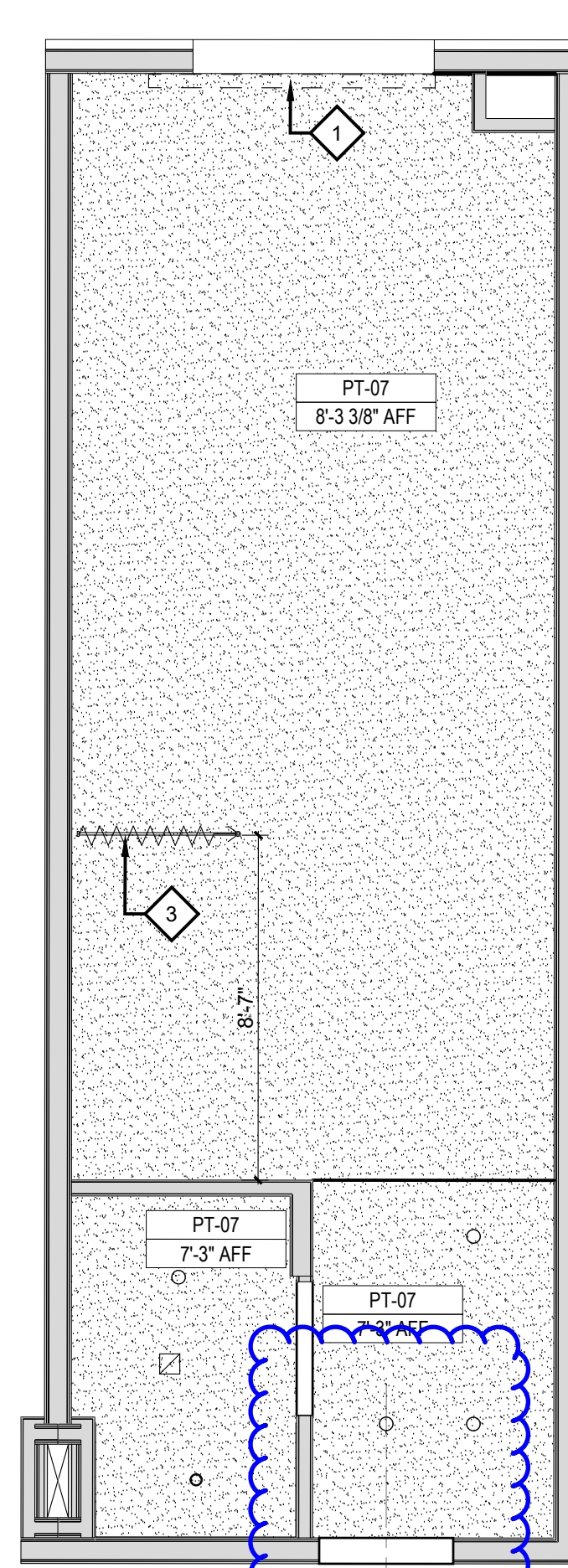
2 RCP PLAN
