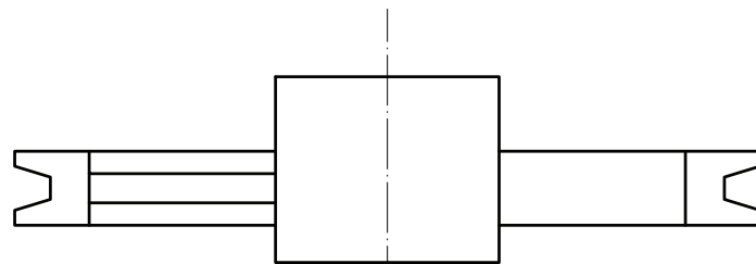
Corte - AB
