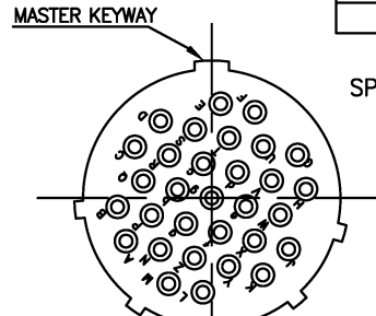
CN3 : 24-31SX (31 #16)
