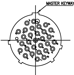
CN1 : 24-31SX (31 #16)
