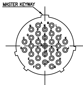
CN4 : 24-31P (31 #16)
