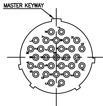
CN5 : 24-31PW (31 #16)
