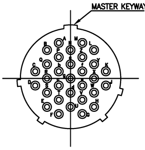
CN2 : 24-31PN (31 #16)
