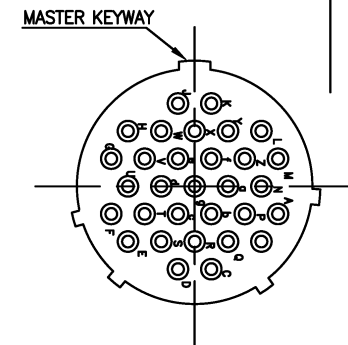
CN2 : 24-31SW (31 #16)
