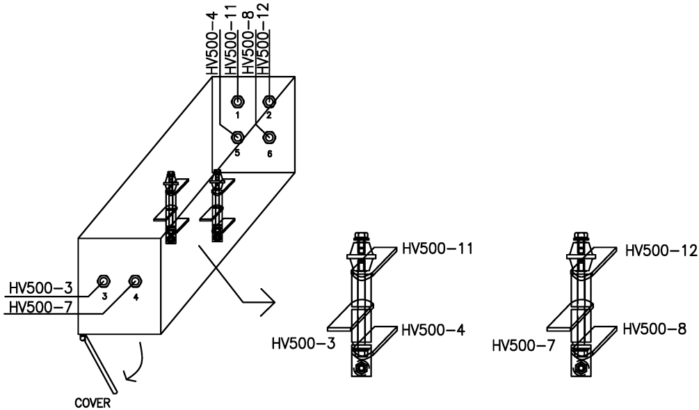
CSJB2 (REAR)
