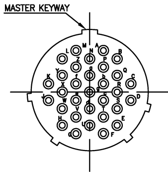
CN1 : 24-31S (31 #16)
