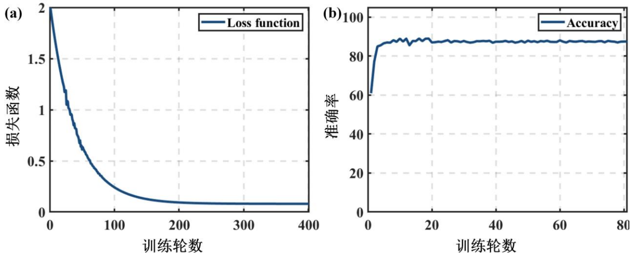
图 34 (a)模型训练的损失函数变化；(b)训练过程中验证集的准确率
