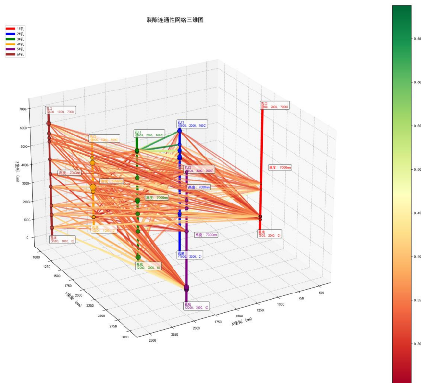
图 4.19 裂隙连通性网络三维图效果图
