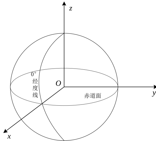
图 2 地心地固坐标系
