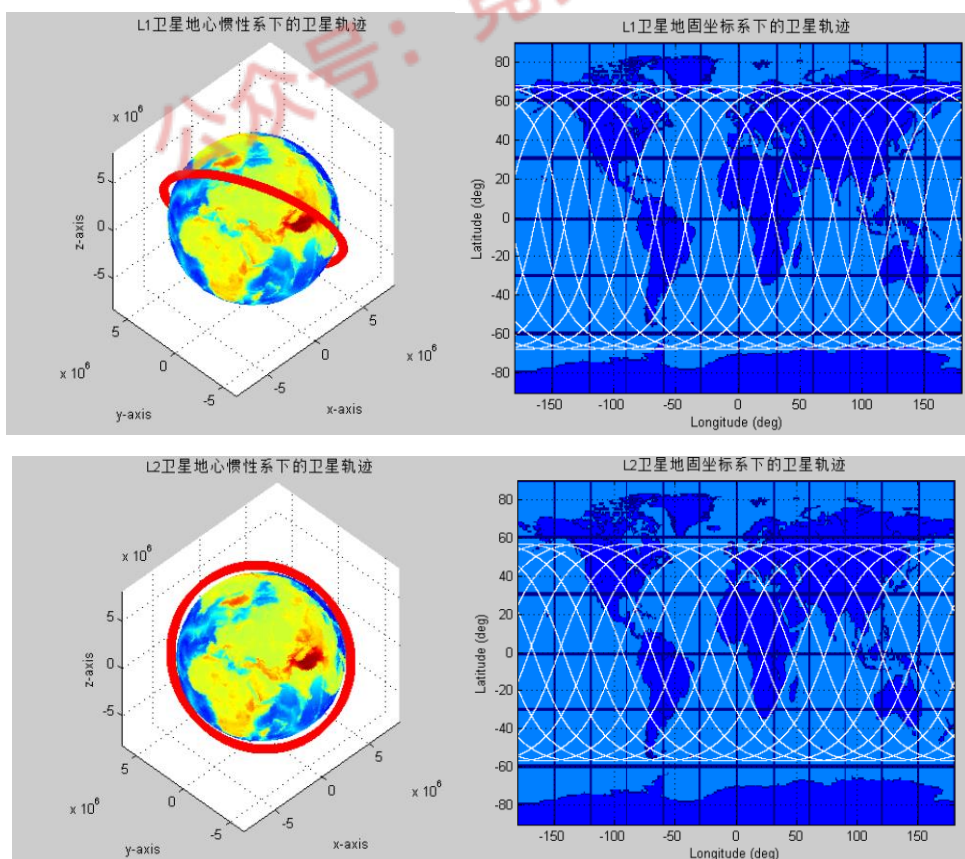
图 11 卫星 L-1 和 L-2 在两个坐标系下的轨迹
