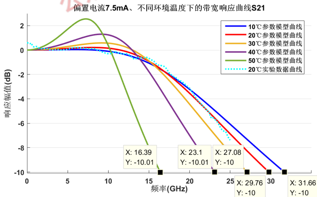
图 3-3 偏置电流 7.5mA、不同环境温度下的带宽响应曲线 S21
