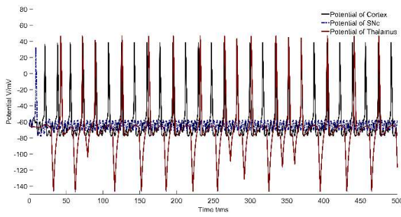
图7.12 CORTEX & THALAMUS 电位变化曲线
