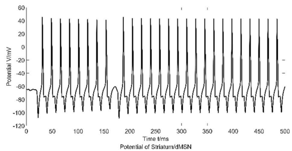
图8.14 dMSN 电位变化曲线
