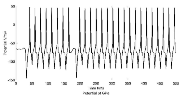
图8.38 GPe 电位变化曲线
