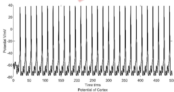
图8.24 Cortex 电位变化曲线
