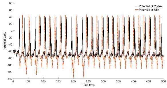
图8.11 Indirect 电位变化曲线
