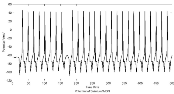
图7.16 iMSN 电位变化曲线
