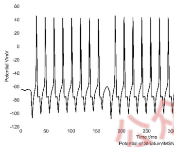
图9.3 iMSN 电位变化曲线
