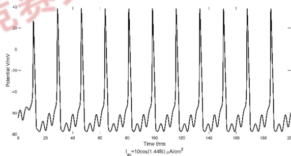
图5.10 交流刺激 ( \omega = 1.448 )
