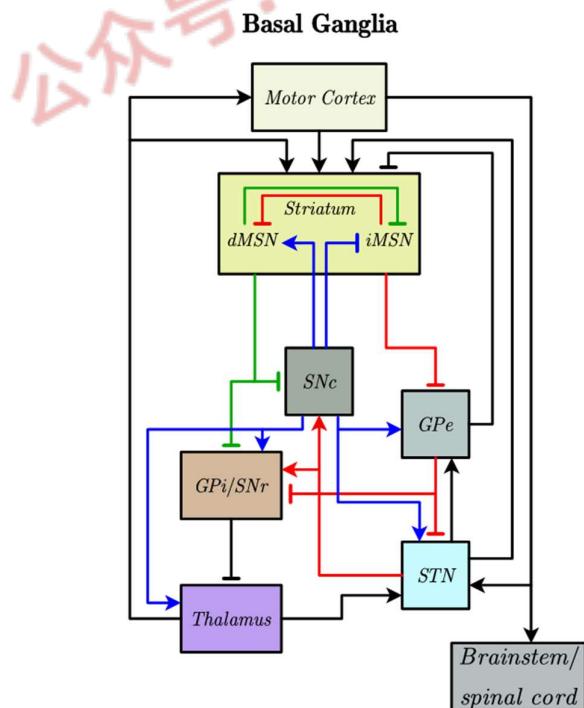
图1.1 基底神经节内部神经核团连接（箭头方向代表兴奋，方块方向表示抑制，绿色路径是直接通路，红色路径是间接通路，蓝色路径是多巴胺）
