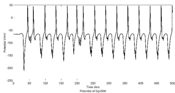
图7.19 GPi-SNr 电位变化曲线
