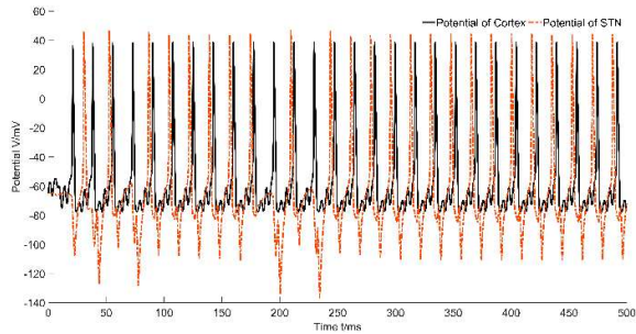
图7.23 Indirect 电位变化曲线
