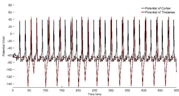
图8.9 Cortex & Thalamus 电位变化对比曲线
