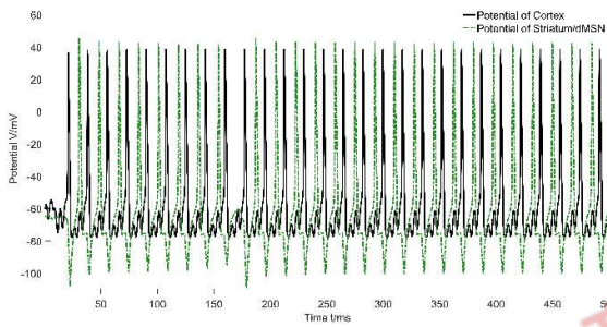
图9.9 Direct 电位变化曲线
