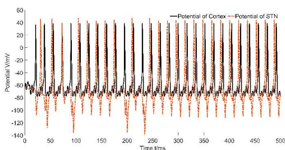
图8.44 Indirect 电位变化曲线
