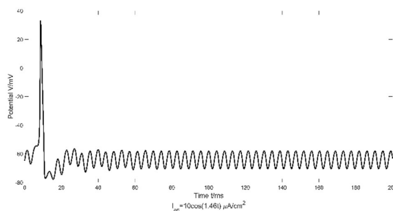
图5.12 交流刺激 ( \omega = 1.46 )
