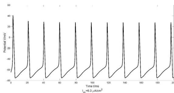
图5.8 直流刺激 6.3 \mu\text{A}/\text{cm}^2
