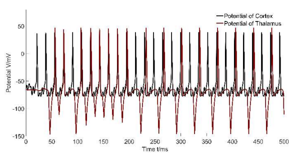
图8.42 Cortex & Thalamus 电位变化对比曲线
