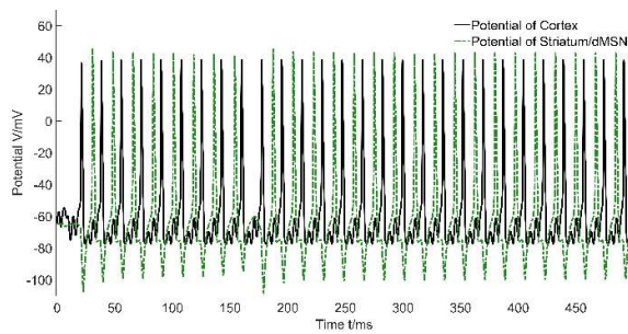
图8.21 Direct 电位变化曲线
