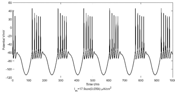
图5.13 交流刺激（幅值为 17.9 \mu A ， \omega = 0.039 ）（左）
