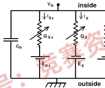
图 3-1 Hodgkin-Huxley 神经元轴突的等效电路
