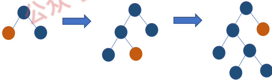
图 5.2 带有深度限制的按叶子生长算法
