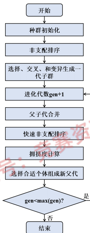
图 5-3 NSGA2 算法流程图
