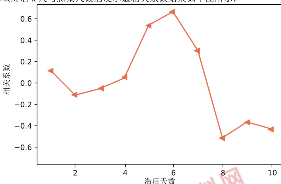
图 4-3 蔬菜出库量滞后 k 天与感染人数的皮尔逊相关系数
