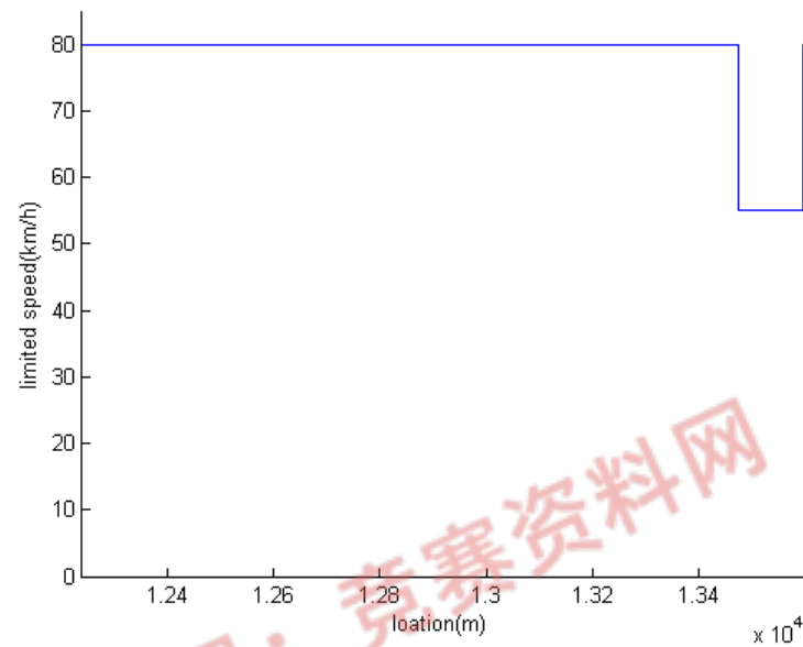
图 5.11 A7-A6 限速图
