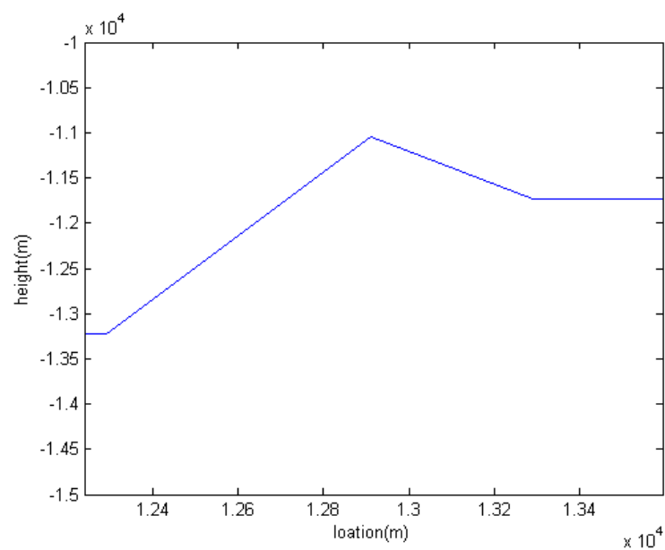
图 5.12 A7-A6 站的坡度
