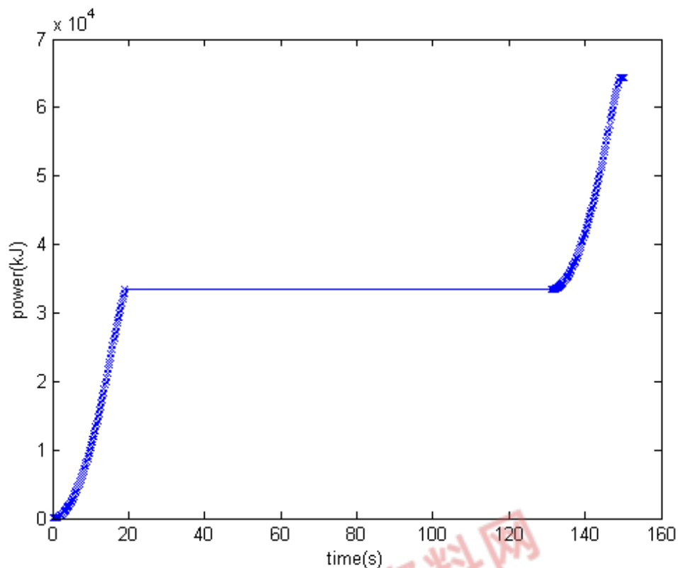
图 5.8 途中有一个车站的单车系统 P-T 图
