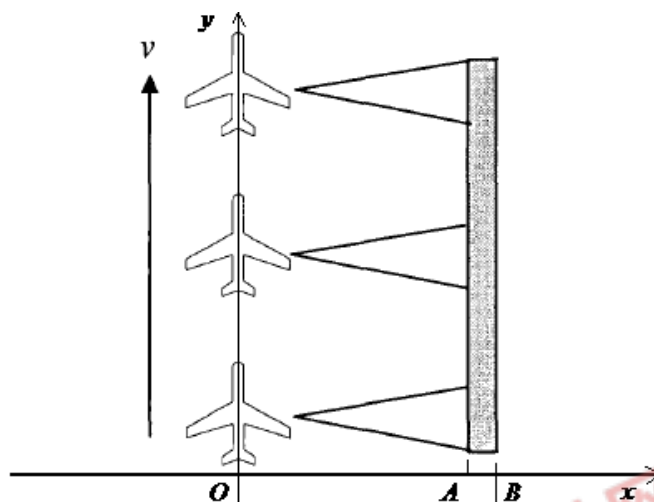
图 4-2 成像传感器工作原理及相关性能参数示意图
