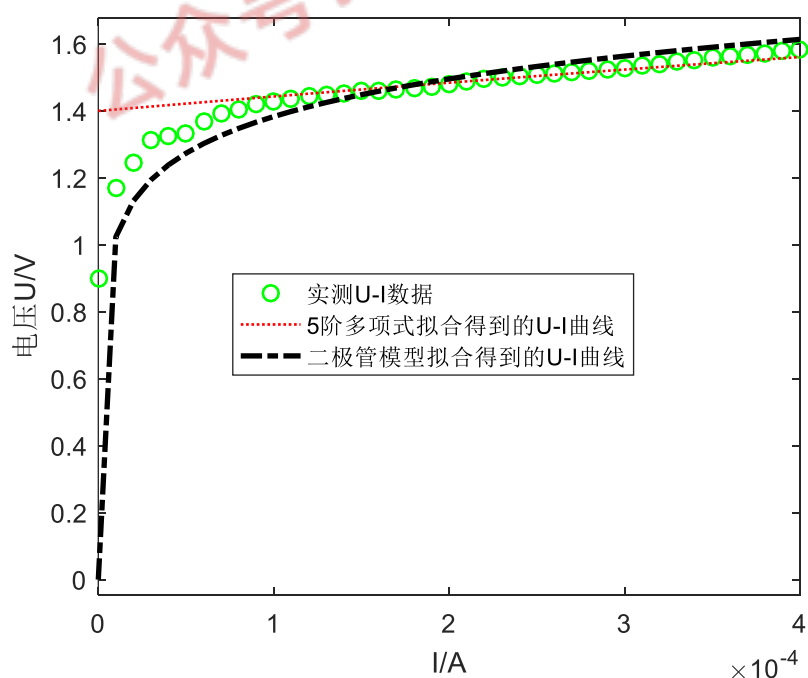
图 11 不同拟合方法电压外推后的曲线局部对比（小电流端）
