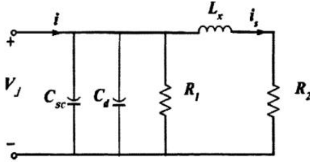
图 27 VCSEL 的本征网络小信号等效电路模型 由电路分析, 可以导出 VCSEL 等效电路的频率响应表达式为:
