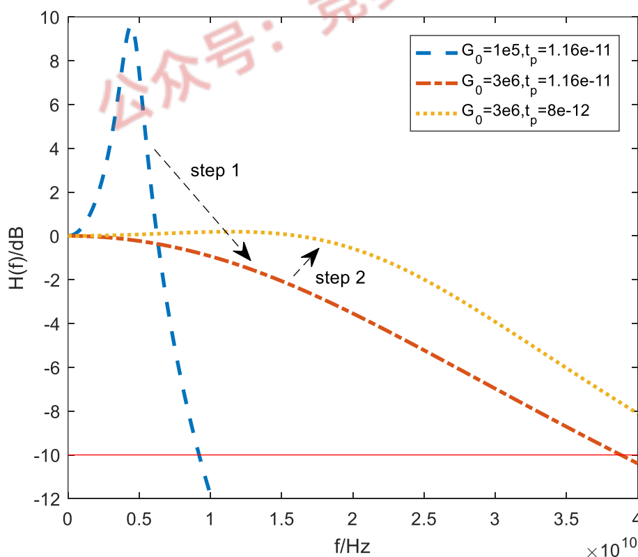
图 26 通带平坦度相关参数调整
