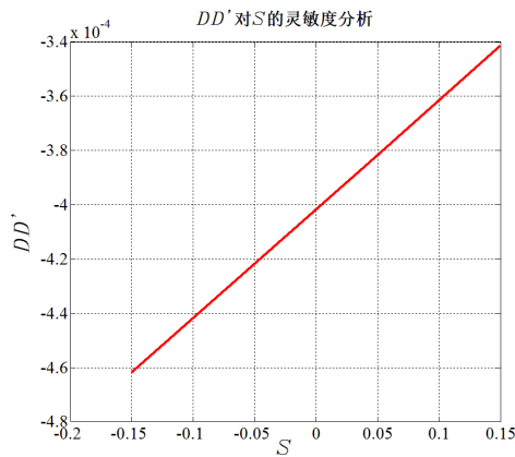
图 30 \Delta T_{air}/T_{air} 、 \lambda 和 DD' 对 S 的灵敏度分析
