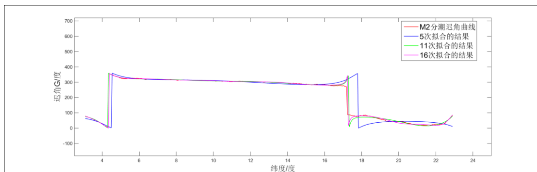
图 5-4 M_2 分潮迟角曲线对比图
