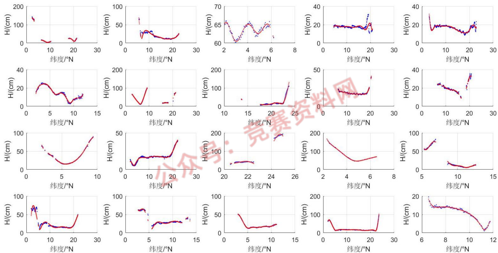
图 4-14 南海区域内 20 条轨道上 M2 正压潮振幅结果图（红色的为正压潮）
