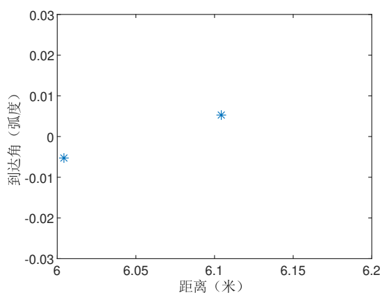
图 4.31 变分贝叶斯线谱估计 MDVALUE 问题四估计结果
