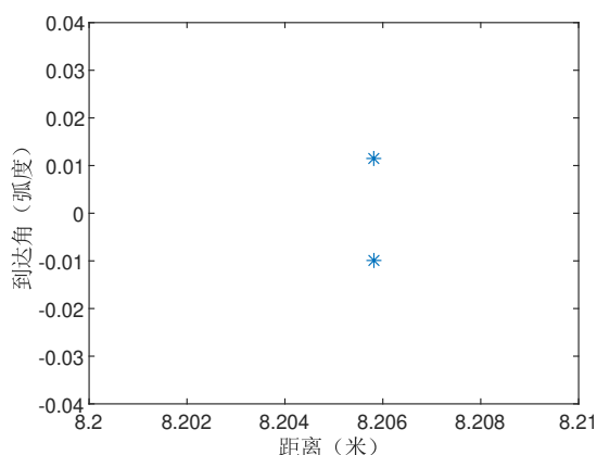
图 4.11 变分贝叶斯线谱估计 MDVALUE 问题二估计结果
