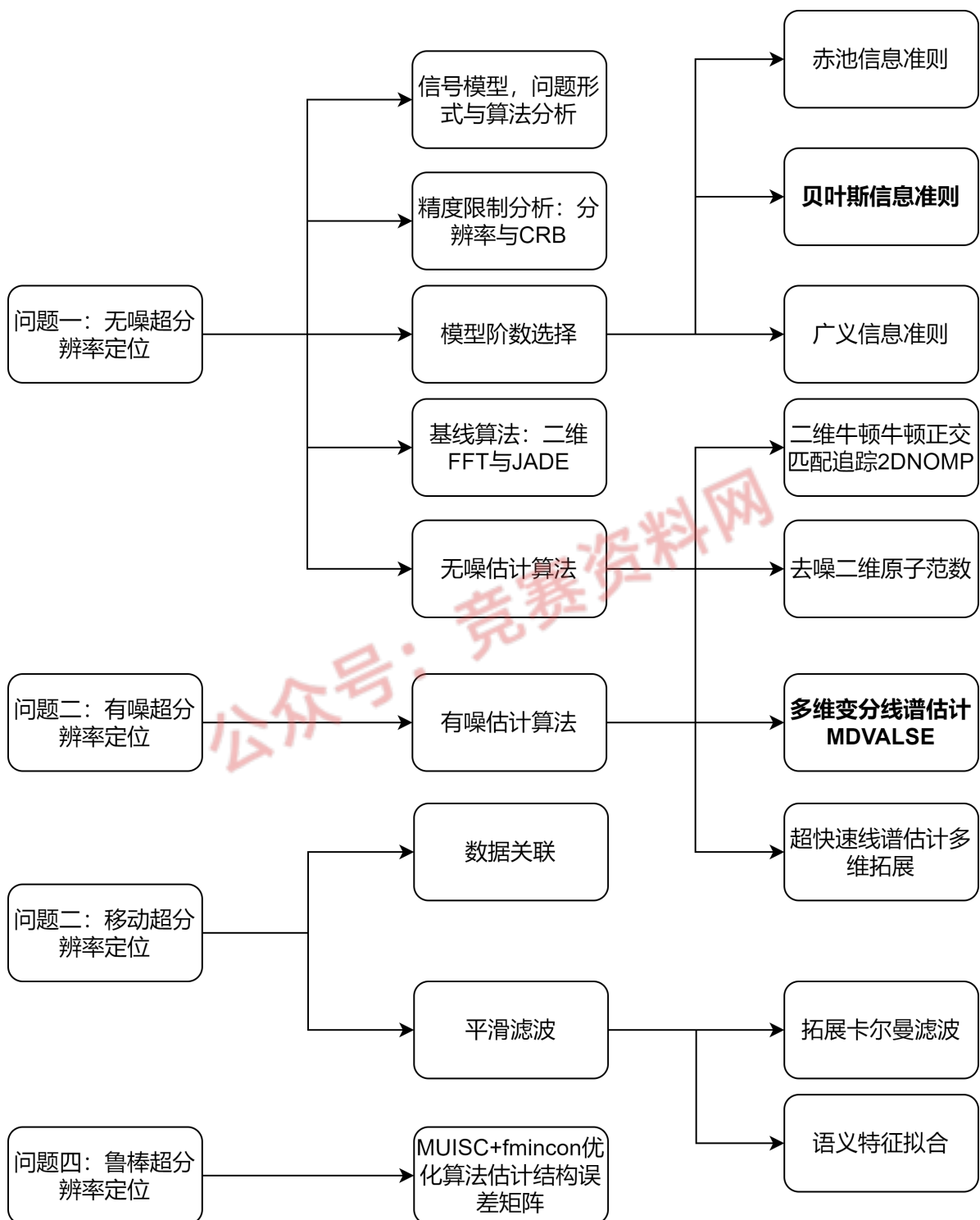
图 1.1 算法框图
