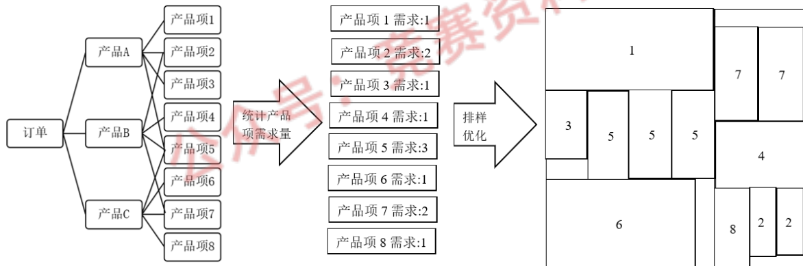
图 1 订单组批与排样优化过程图
