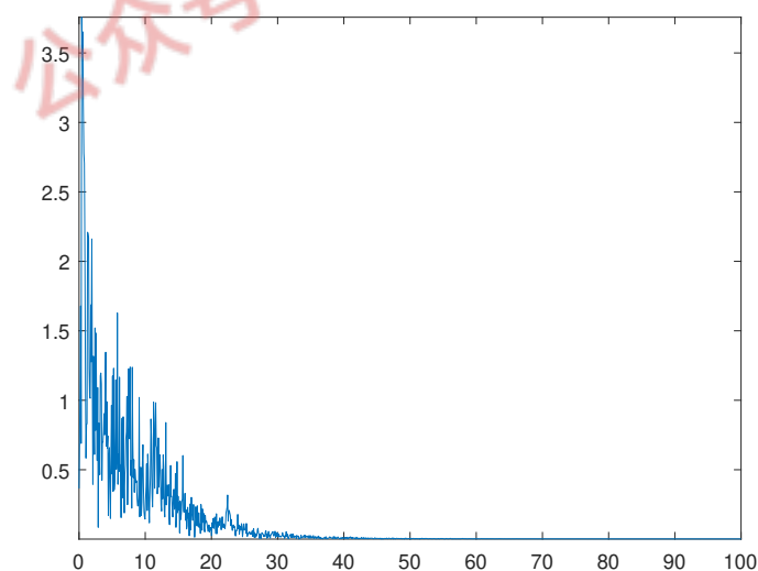
图 4-12 滤波后字符 char14 通道 1 的数据频谱
