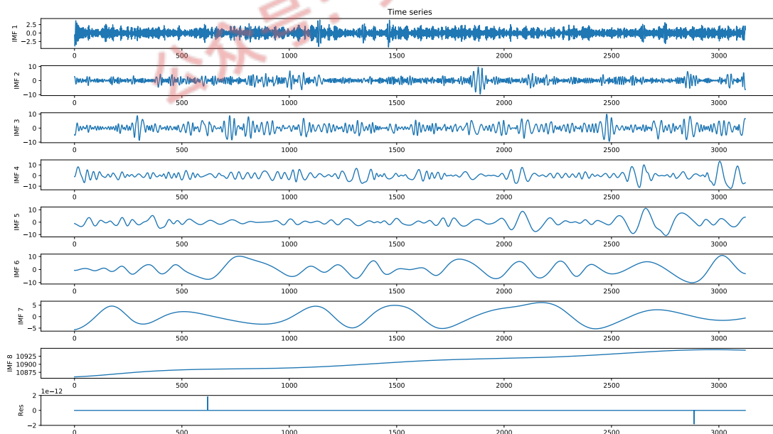
图 4-2 EMD 分解字符 char01(B) 通道 1 得到的 IMF 分量
