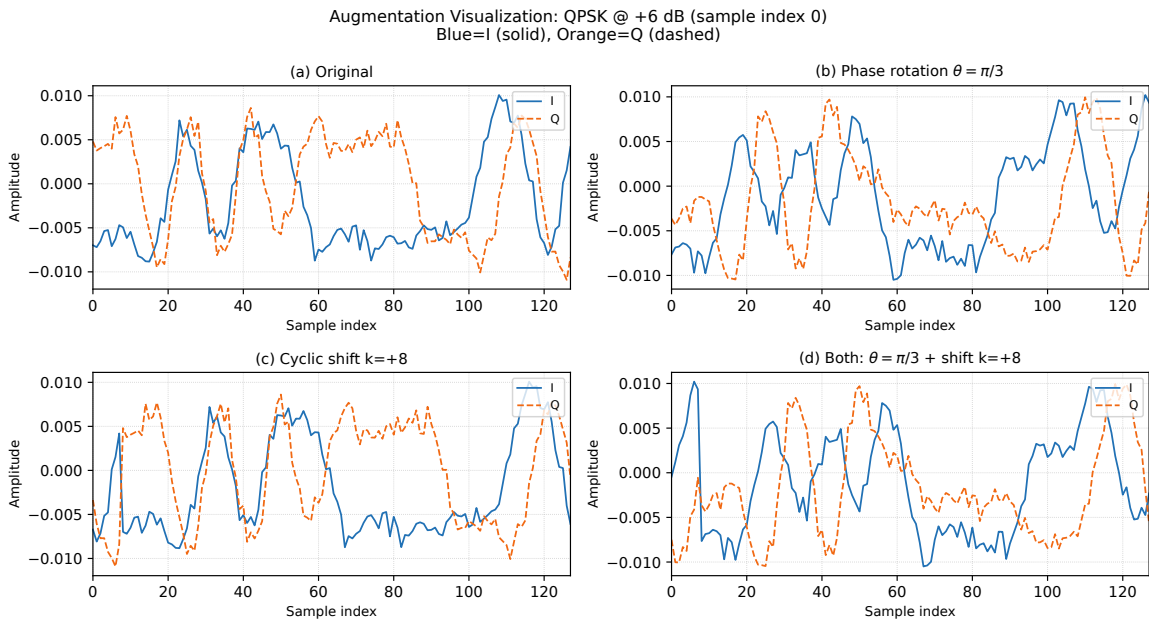
图 3.3 信号域增强示例（QPSK @ +6 dB 单样本）。(a) 原始；(b) 相位旋转 \theta = \pi/3 ；(c) 循环时移 k = +8 ；(d) 两者叠加。I/Q 通道线型见图例。
