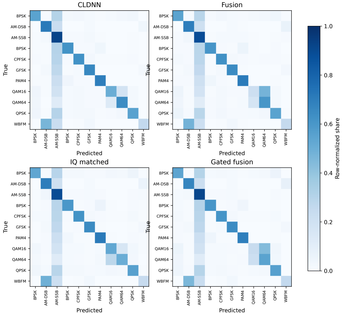
图 A.2 代表模型在 overall scope 下的行归一化混淆矩阵,三训练种子聚合。Data source: confusion_overall.csv for seeds 42, 2025, and 3407.
