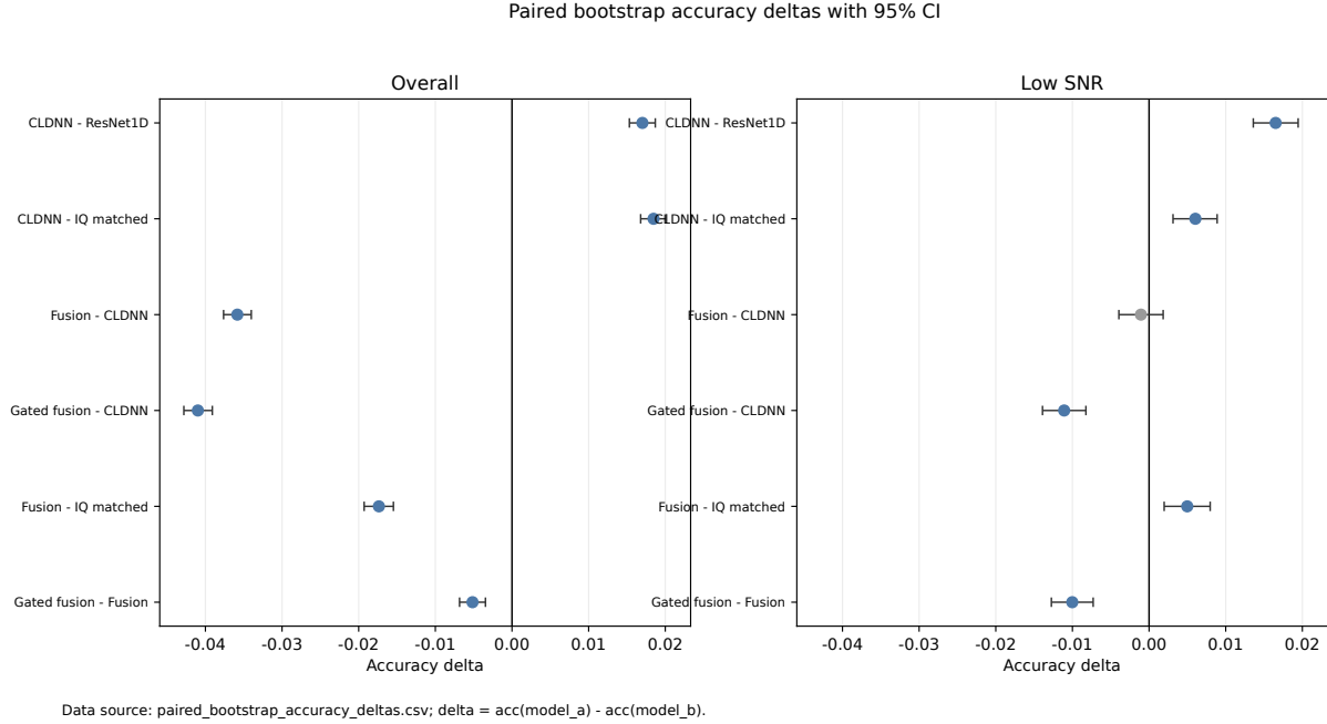
图 4.4 已登记 paired bootstrap accuracy delta 及其 95% 置信区间。Data source: paired_bootstrap_accuracy_deltas.csv; delta = \text{Acc}(m_a) - \text{Acc}(m_b) 。
