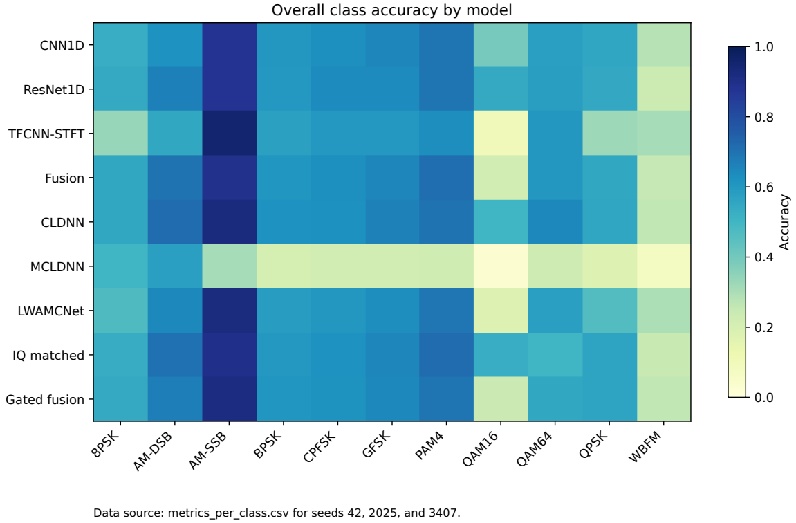
图 4.3 9 个模型行在 11 类调制方式上的 overall class accuracy。Data source: metrics_per_class.csv for seeds 42, 2025, and 3407.
