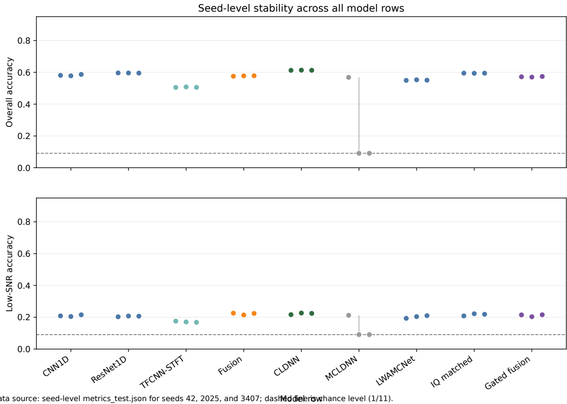
图 4.9 9 个模型在 3 个训练种子上的整体与低信噪比准确率稳定性散点（metrics_test.json）。
