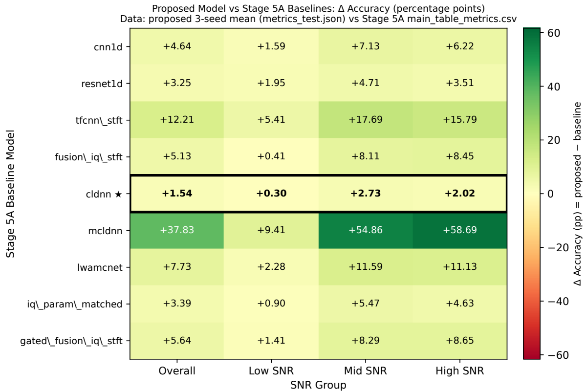
图 4.10 提案模型相对 Stage 5A 九个基线在四个指标（Overall / Low / Mid / High SNR）上的准确率增量热力图（单位：百分点；绿色正增量，红色负增量；行为 CLDNN 基线加粗边框；数据源：三种子均值 metrics_test.json vs main_table_metrics.csv）。
