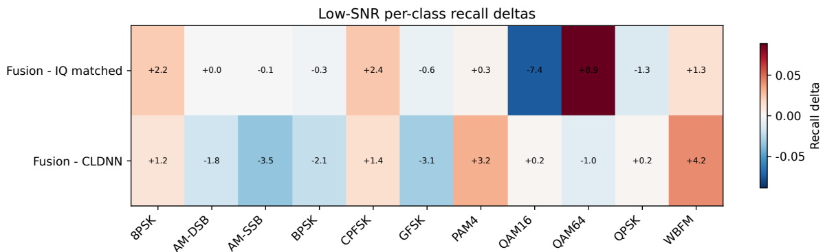
图 4.7 静态 fusion_iq_stft 相对 iq_param_matched 与 CLDNN 在低 SNR 各调制类别的召回率差值 \Delta\text{recall} （confusion_low_snr.csv 三种子聚合）。
