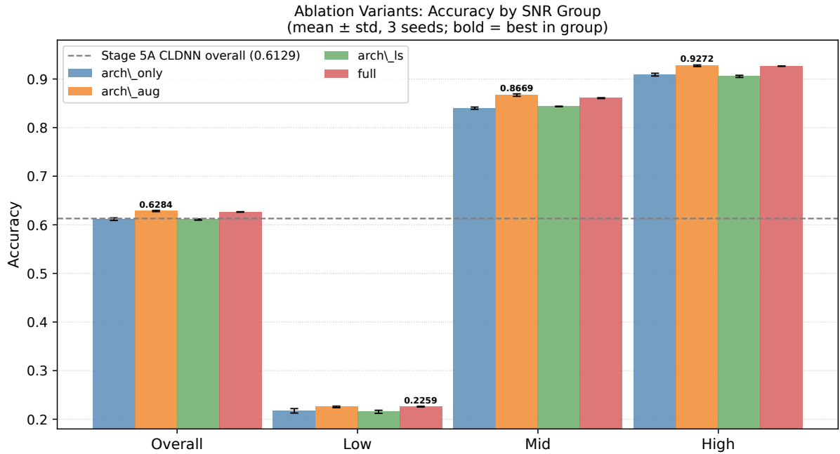
图 4.12 四个消融变体（ arch_only / arch_aug / arch_ls / full ）在 Overall / Low / Mid / High SNR 分组上的准确率均值 \pm 标准差（三种子，数据源： metrics_test.json ）。每柱顶标注该分组最优值（加粗），水平虚线 = Stage 5A CLDNN 整体基线（0.6129）。
