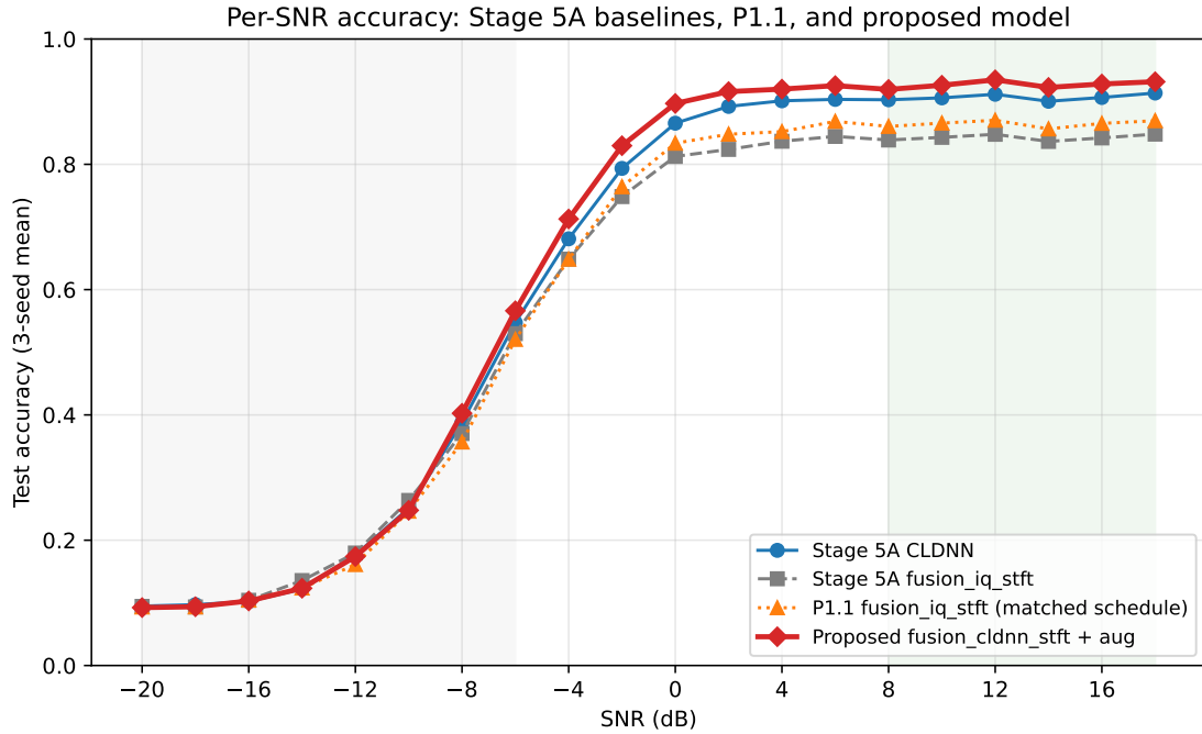
图 4.11 提案模型与三类对照的逐 SNR 准确率曲线（三训练种子均值）。灰/绿阴影区分别为低 SNR ( \leq -6 dB) 与高 SNR ( \geq 8 dB) 范围。
