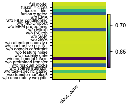
B R2 per variant
