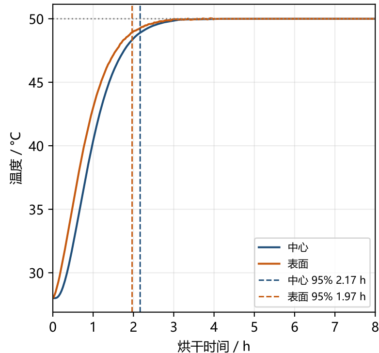
(a) 预热阶段温升 (问题二轨迹)
