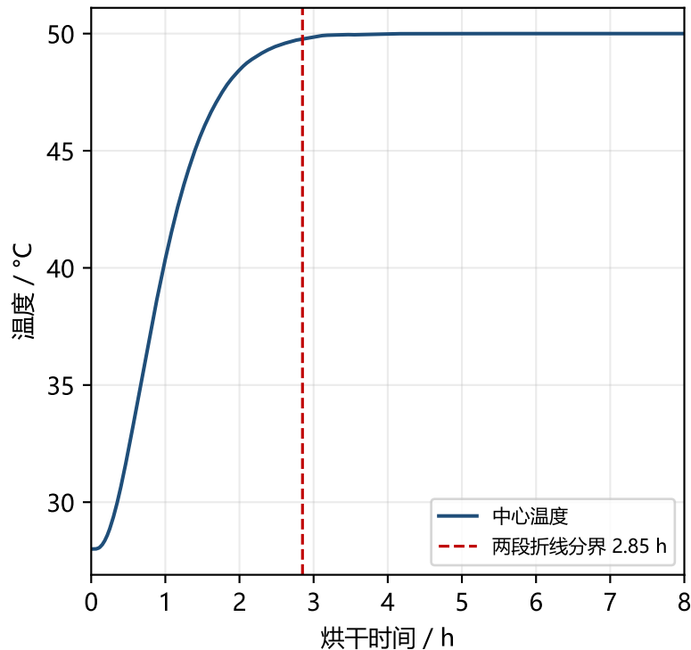
(b) 两段折线回归分界
