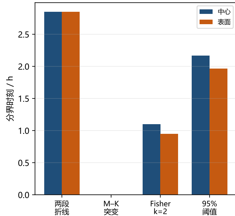
(c) 四种方法的分界时刻对照
