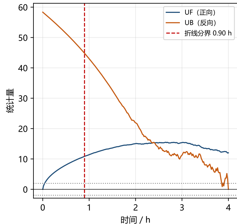
(a) 烘房温度的 M-K 突变检验与折线分界
