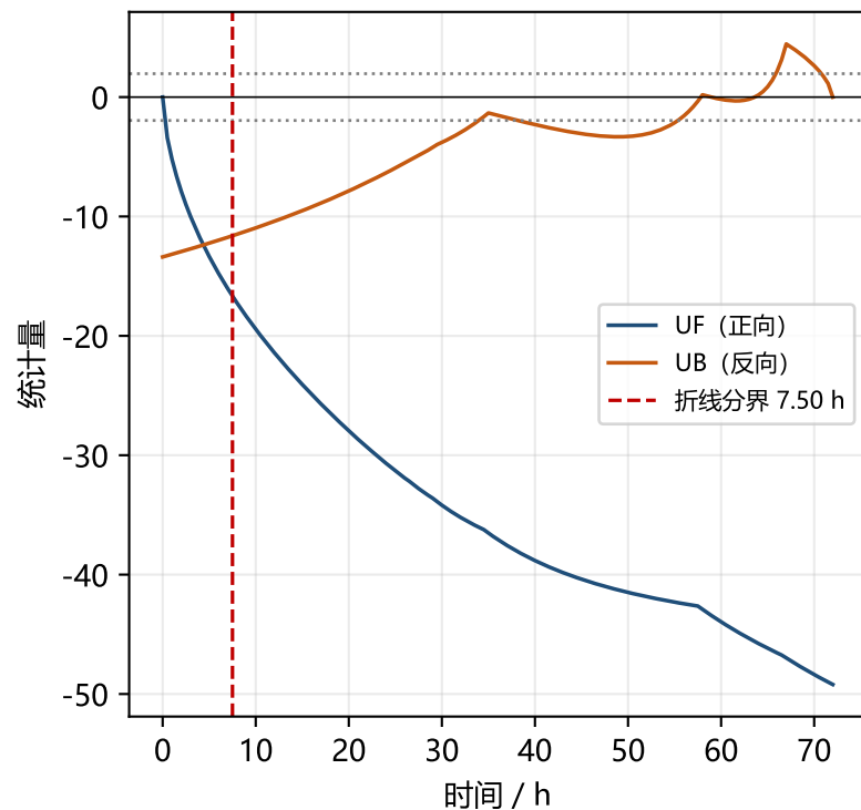
(c) 药材半径的 M-K 突变检验与折线分界
