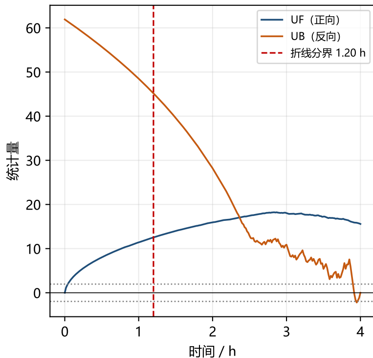
(b) 烘房水分指标的 M-K 突变检验与折线分界
