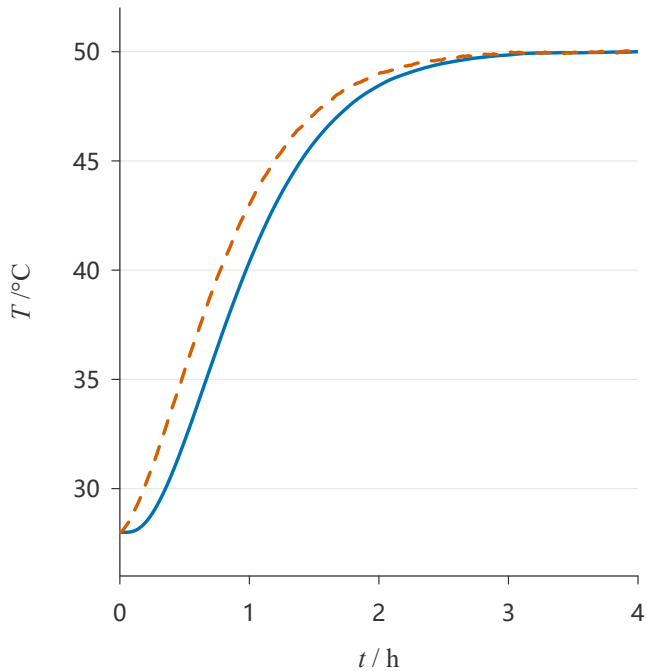
(a) 前 4 h 的温度响应
