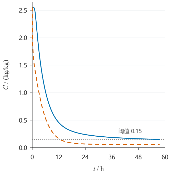
(b) 全过程干基含水率
