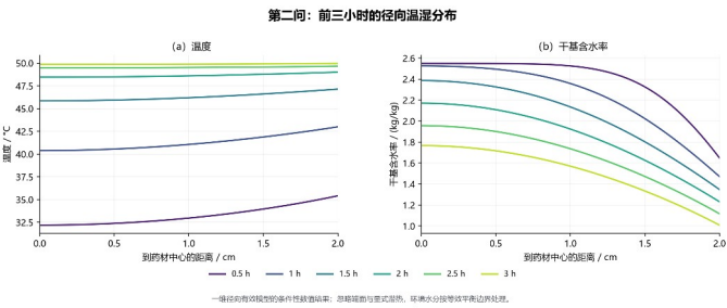
图 5 问题二 3 h 内的径向温湿剖面:(a) 温度(°C)与 (b) 干基含水率(kg/kg)随到中心距离(cm)的分布;曲线对应 0.5—3.0 h,温度趋于均匀而含水率仍保持梯度。
