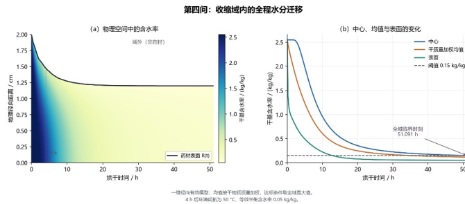
图 7 问题四的全域水分迁移:物理空间含水率(kg/kg)随烘干时间(h)与径向距离(cm)的分布,以及材料点含水率随时间的演化;标注全域临界时刻 51.0906 h。
