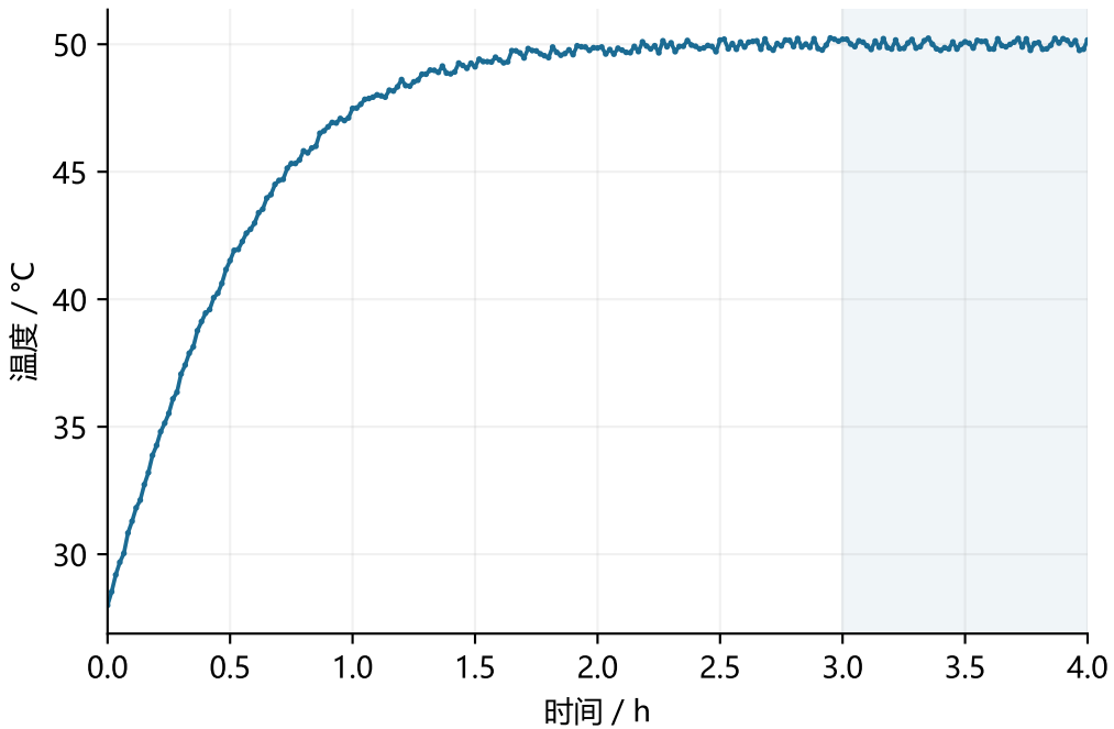
烘房温度
