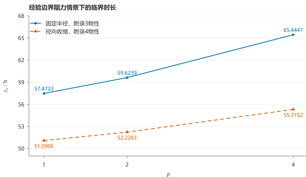
图 6 经验边界阻力参数对临界烘干时长的影响 ( N=800 )
