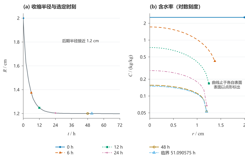
图5 问题四半径收缩过程与域内干基含水率分布
