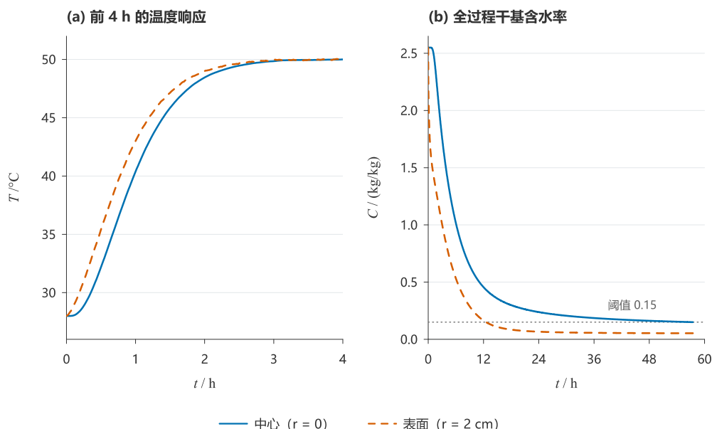
图 3 问题二中心与表面的温度及干基含水率变化
