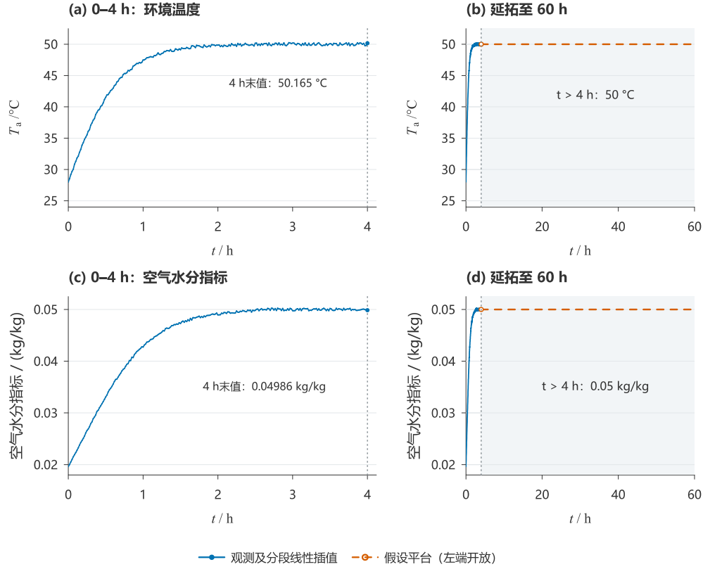
图2 烘房温度与空气水分指标的观测插值及平台延拓
