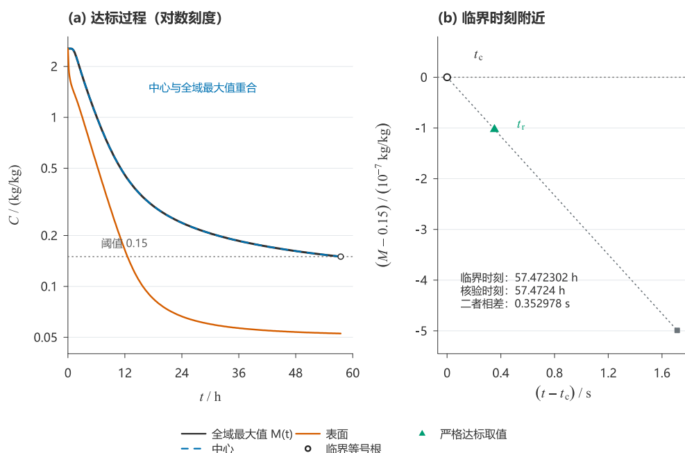
图4 问题三全域含水率达标过程及临界时刻局部放大
