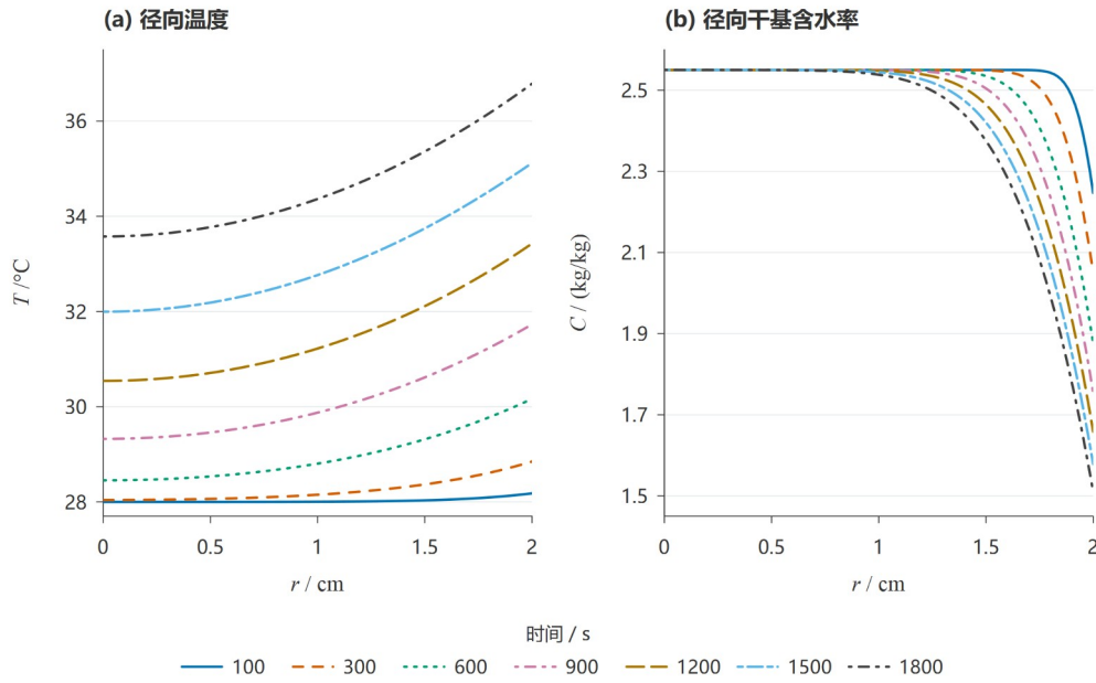
图1 问题一不同时刻的径向温度与干基含水率分布
