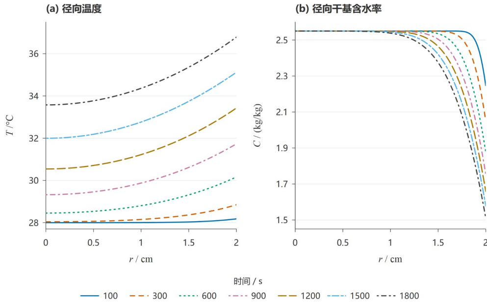
图1 问题一不同时刻的径向温度与干基含水率分布
