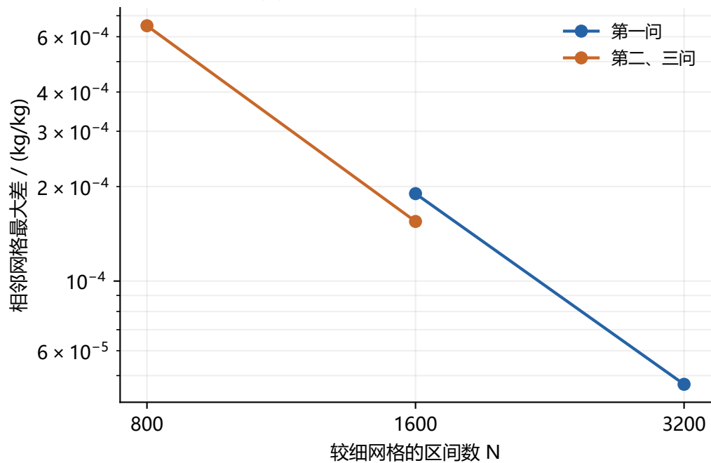
(a) 共同物理采样点的最大含水率差
