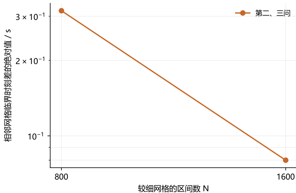
(b) 全域临界时刻的变化
