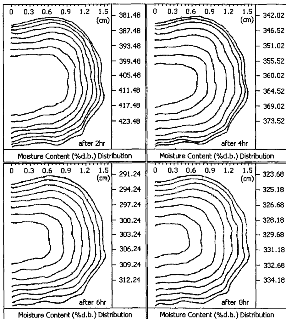
图 4.17 地黄预测含水率分布图
