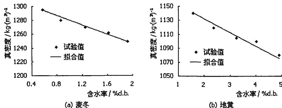
图 3.6 真密度与含水率的关系
