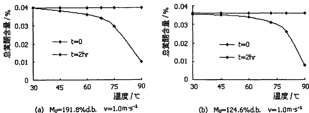
图 2.17 风温对麦冬总黄酮含量的影响
