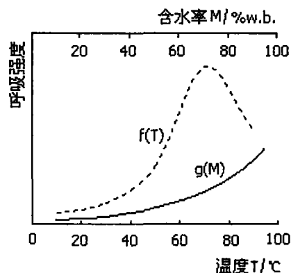
图 2.1 呼吸强度曲线图
