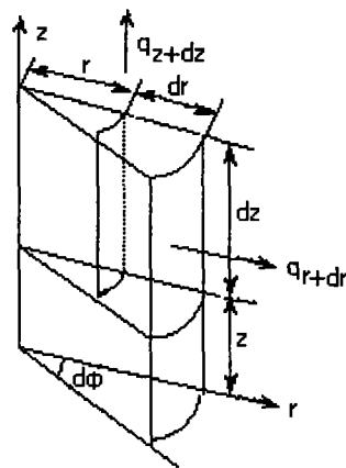
图 4.1 圆柱坐标下微元体热量分析
