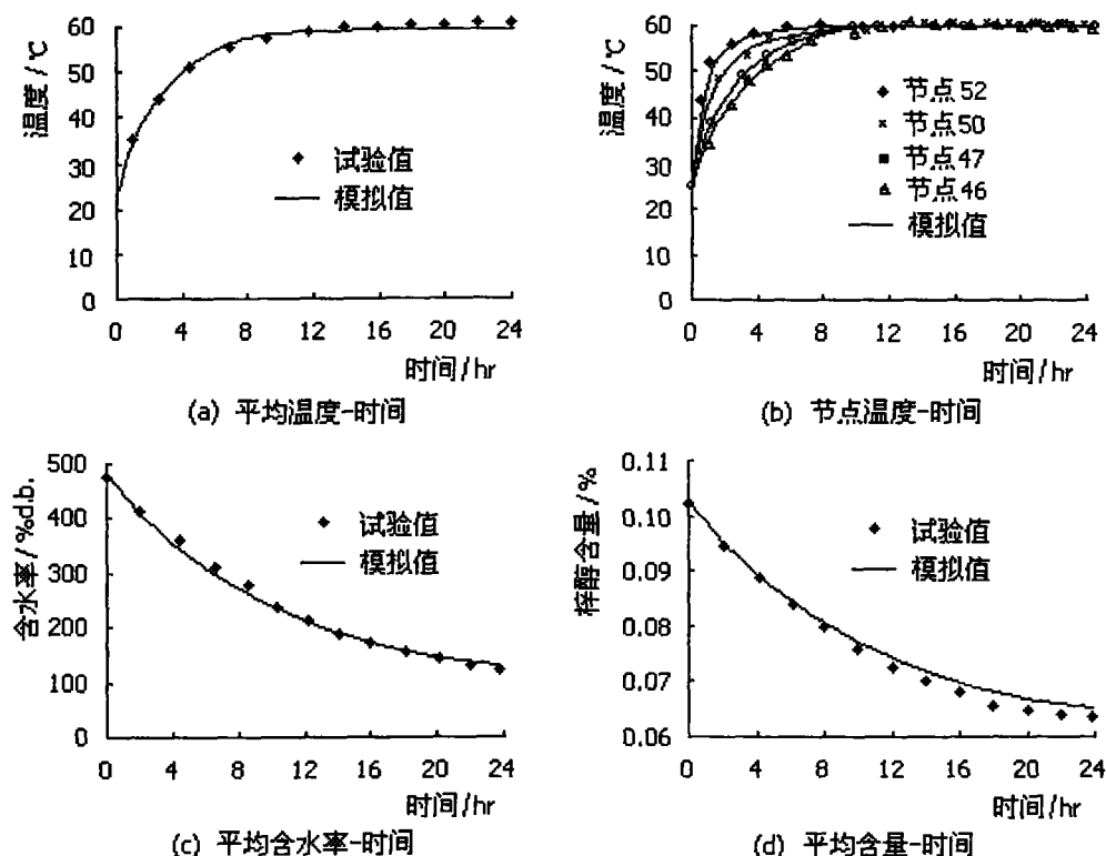
图 4.15 地黄试验值与模拟值的比较
