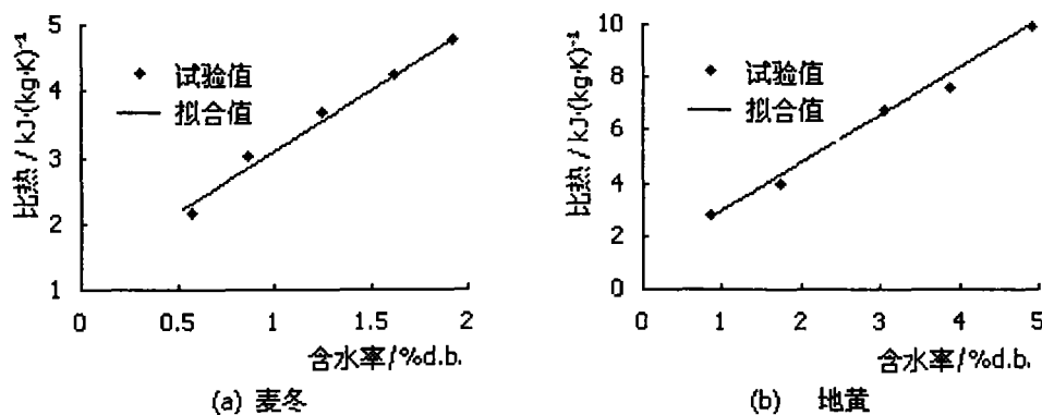
图 3.7 比热随含水率变化图
