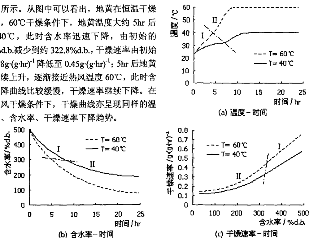
图 5.1 地黄干燥曲线模拟图
