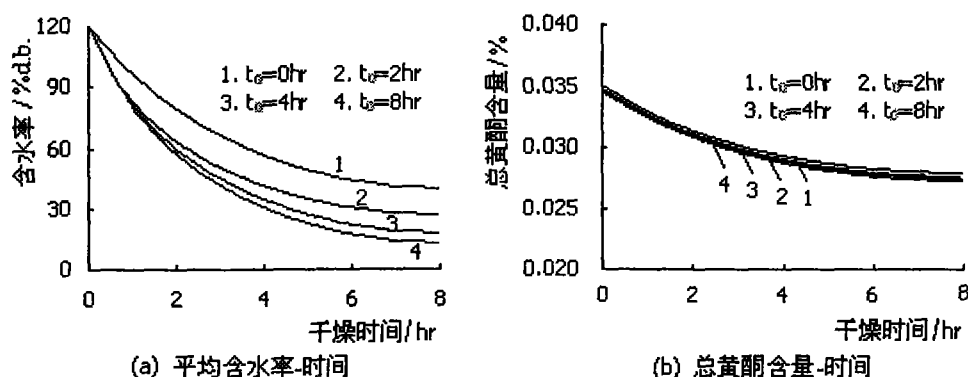
图 5.9 发汗时间对麦冬二次干燥的影响
