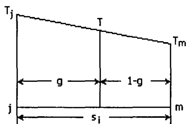
图 4.5 边界插值函数的确定
