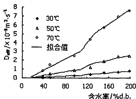
图 3.4 地黄水分扩散系数与含水率的关系
