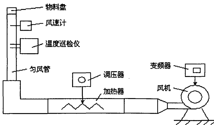
图 2.10 薄层干燥试验装置示意图
