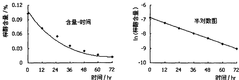
图 2.20 地黄梓醇含量变化图 (70℃水浴)
