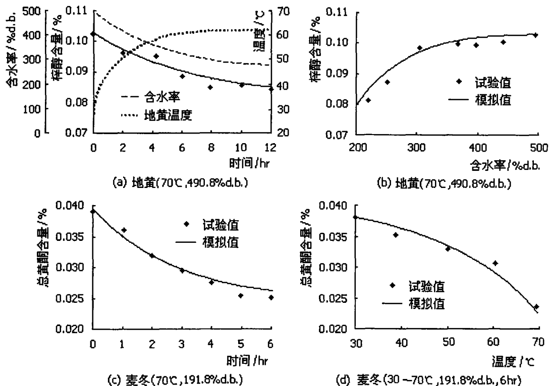
图 2.22 质量退化试验值和模拟值的比较
