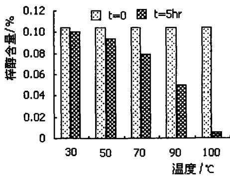
图 2.11 风温对梓醇含量的影响
