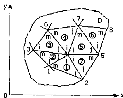
图4.3 平面划分为三角形单元
