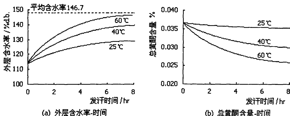
图 5.7 发汗温度对麦冬发汗过程的影响
