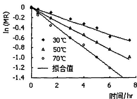
图 3.3 地黄 \ln MR 与时间的关系图
