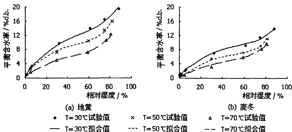
图 3.1 中药材等温解吸曲线图
