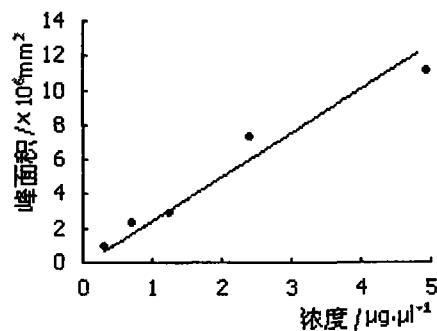
图 2.8 梓醇标准曲线
