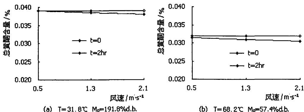
图 2.19 风速对麦冬总黄酮含量的影响
