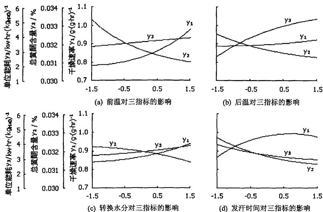
图 5.10 各因素对三指标的影响
