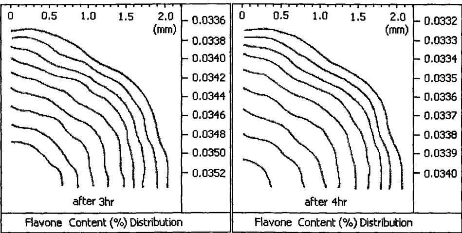
图 4.13 麦冬总黄酮预测含量分布图
