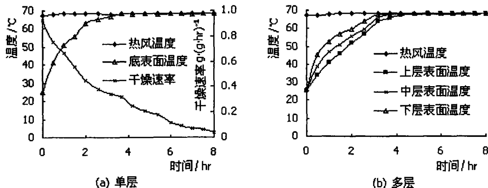
图 3.2 麦冬温度及干燥速率曲线
