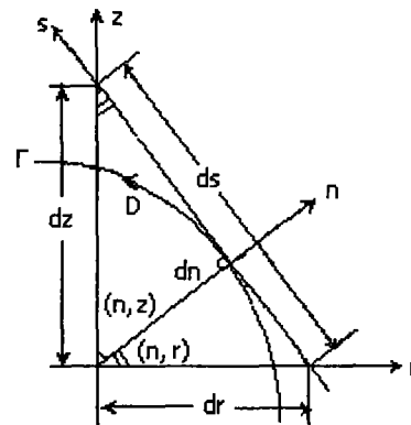
图 4.2 边界坐标与方向余弦
