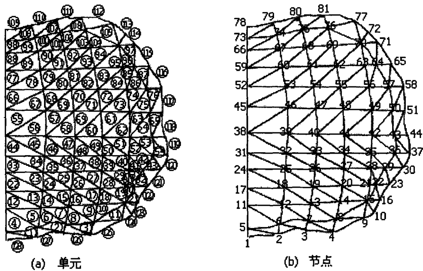
图 4.14 地黄 1/2 截面被剖分为 128 个单元及 81 个节点
