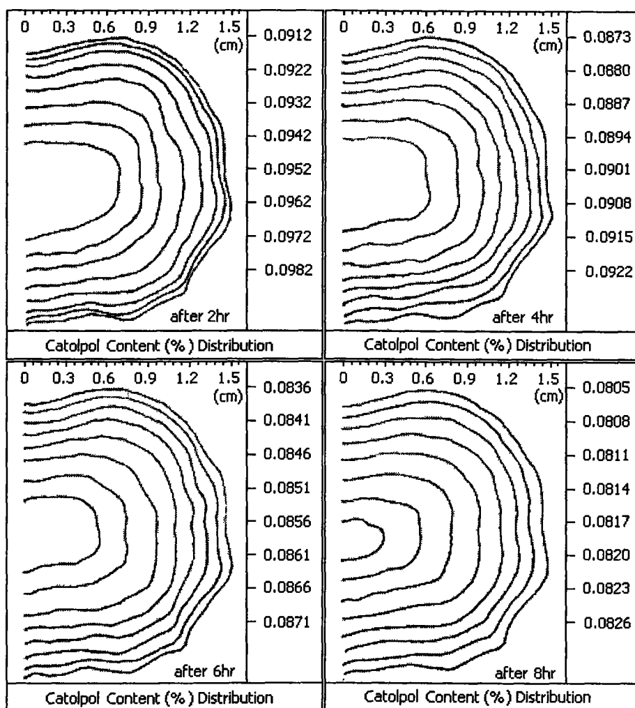
图 4.18 地黄梓醇预测含量分布图
