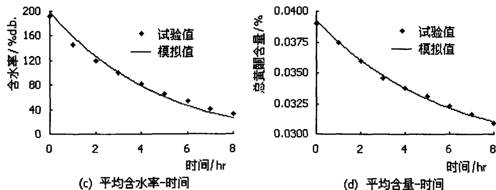
图 4.10 麦冬试验值与模拟值的比较
