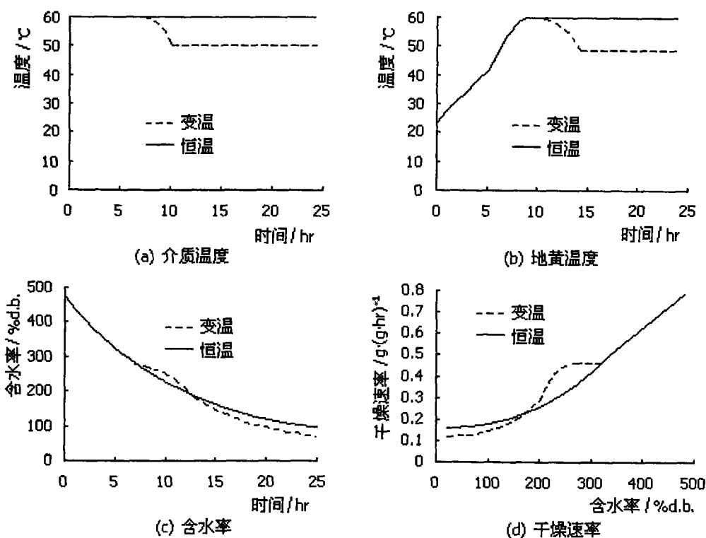
图 5.5 地黄变温干燥曲线图
