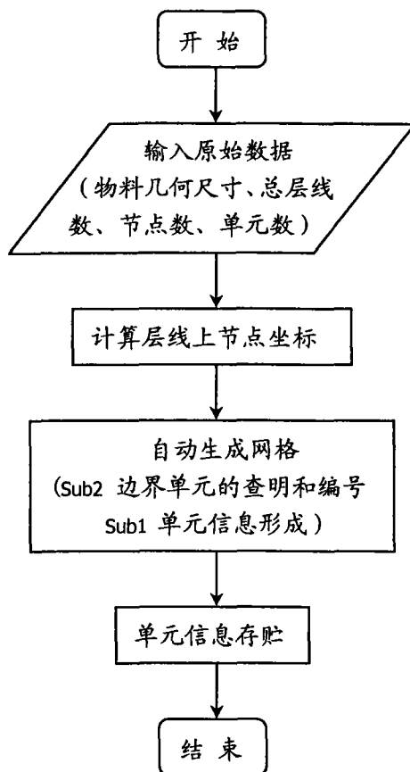
图 4.6 有限单元网格自动生成程序结构图
