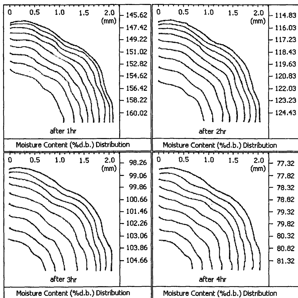
图 4.12 麦冬预测含水率分布图
