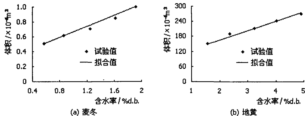
图 3.5 体积与含水率的关系
