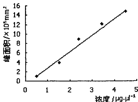
图 2.16 橙皮甙标准曲线
