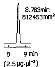
图 2.15 橙皮甙色谱图 图 2.15 表示浓度为 2.5 \mu\text{g}\cdot\mu\text{l}^{-1} 的橙皮甙标样溶液进样 10 \mu\text{l} , 在保留时间为 8.783 分钟时, 出现橙皮甙峰面积为
