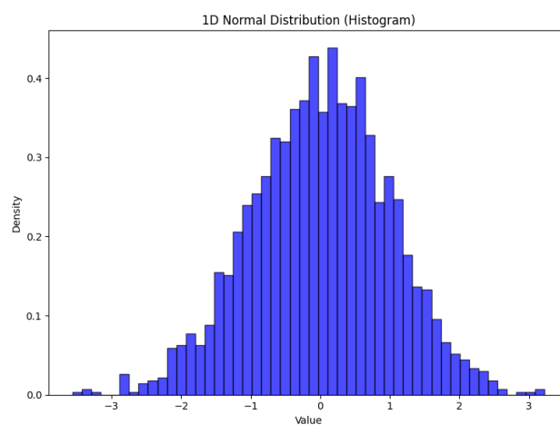
図 1 正規分布に従って生成された数の分布
