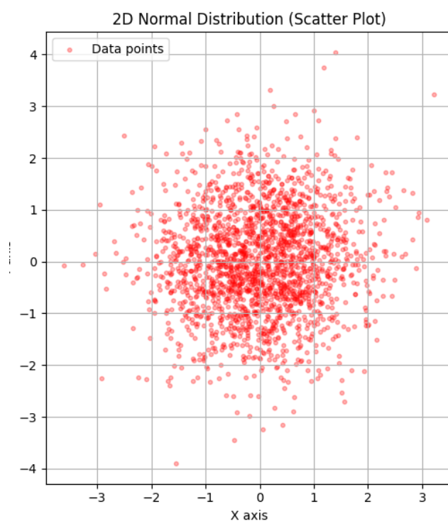
図 2 2次元ブラウン運動の最終時刻における散布図
