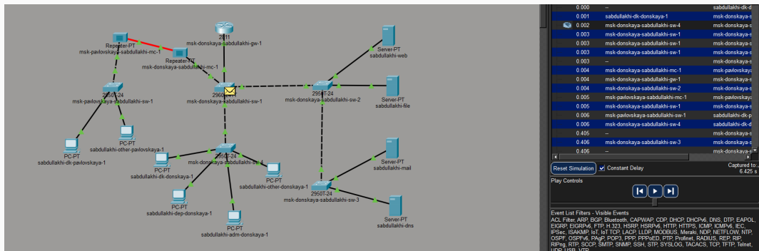
Рис. 13: Процесс обмена DHCP-сообщениями в режиме симуляции
