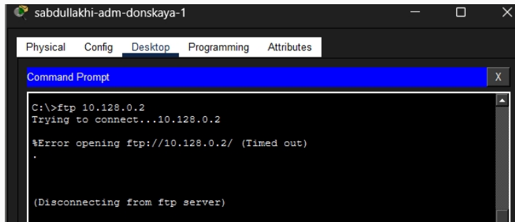
Рис. 9: Запрет FTP-доступа для других пользователей
