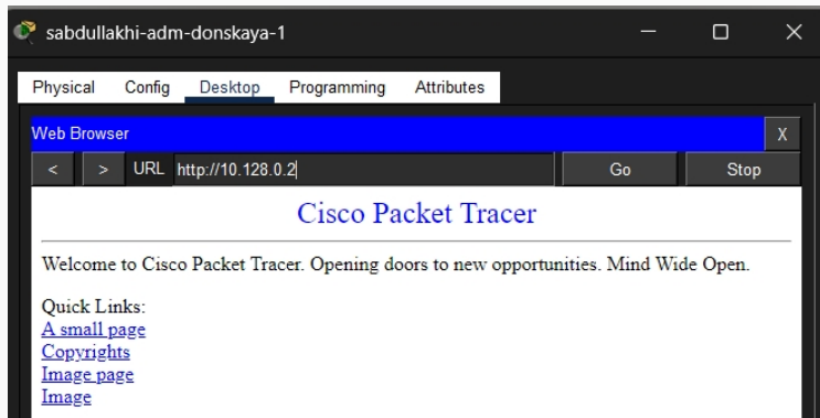
Рис. 4: Проверка HTTP-доступа
