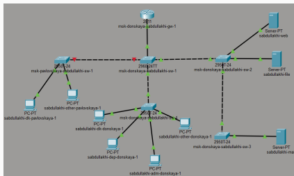
Рис. 10: Отсутствие соединения между коммутаторами
