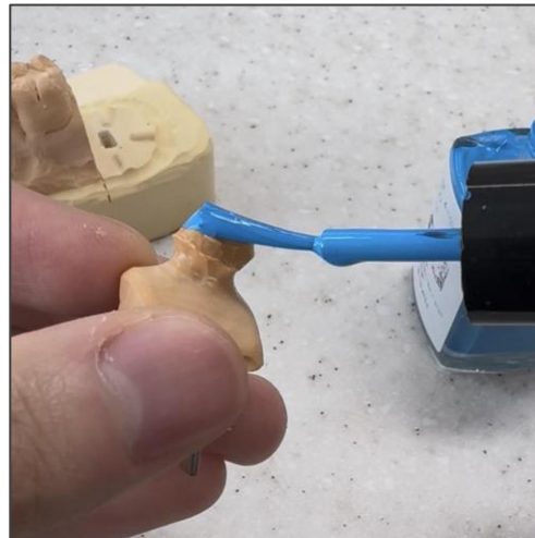
Die Spacer
