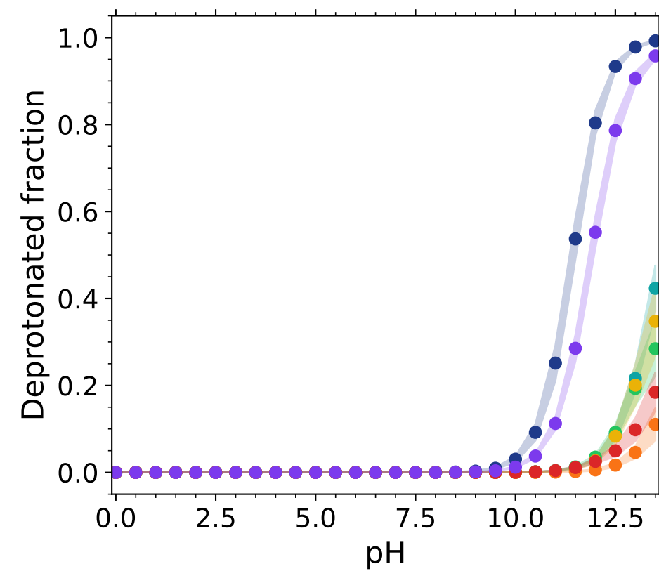
Tyr B:26
