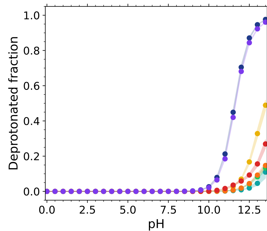
Glu B:13
