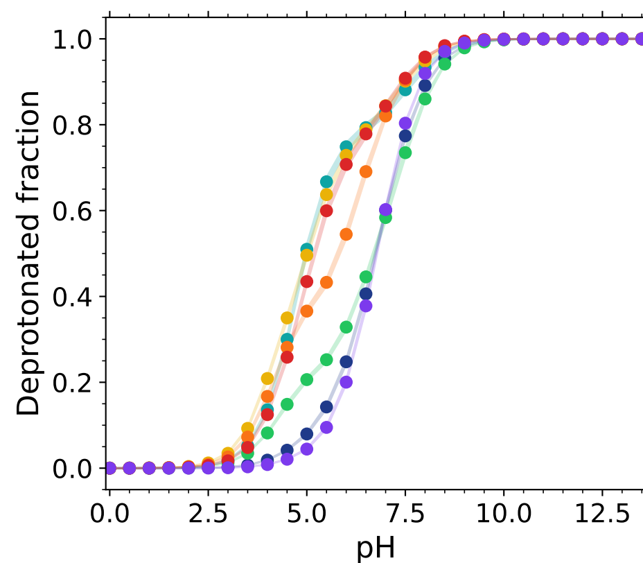
Glu B:21
