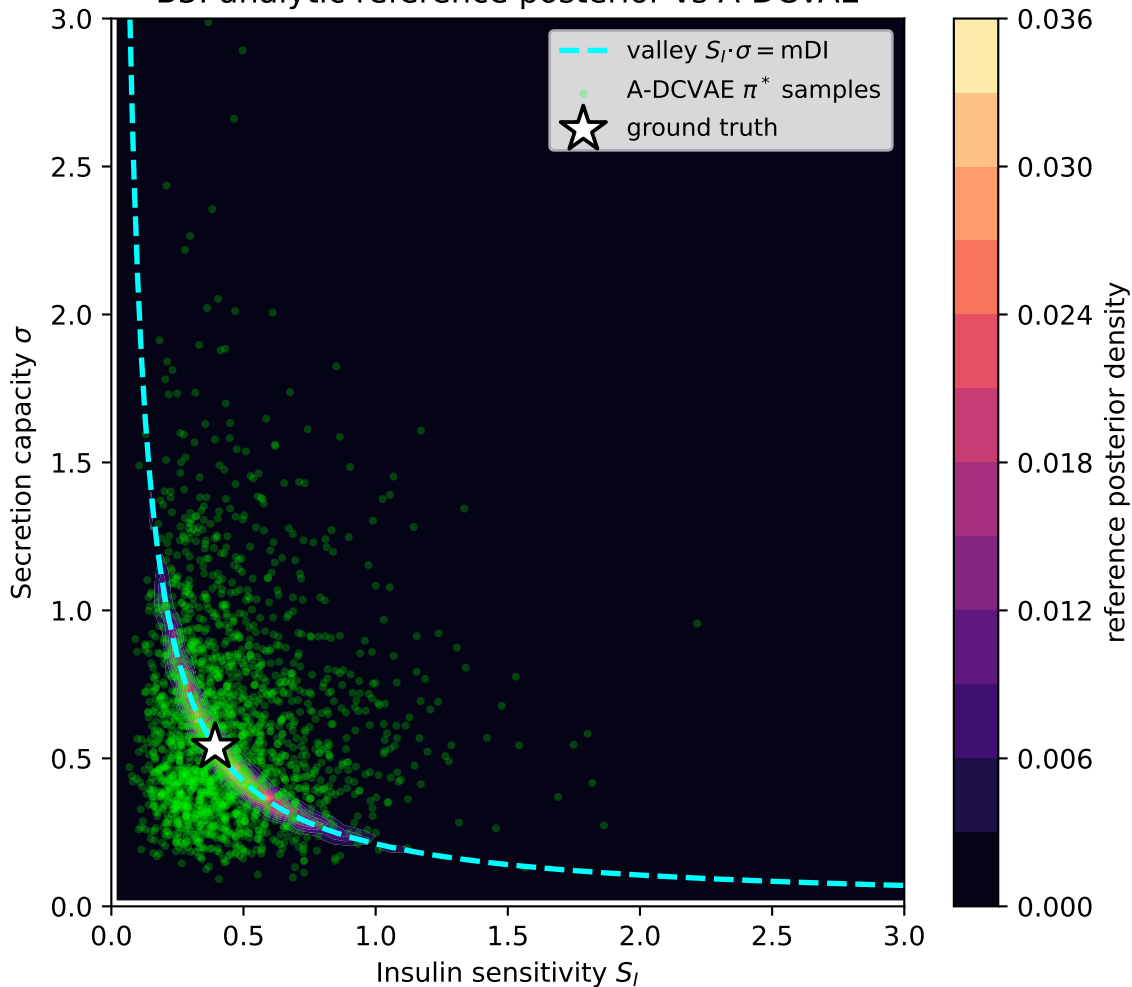
B3: analytic reference posterior vs A-DCVAE
