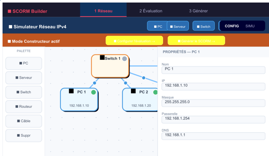
Vue de l'onglet 1 : palette d'appareils, canevas de conception et panneau de propriétés.
