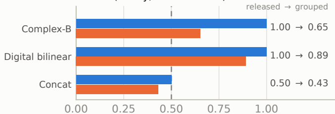
Task B (binary; chance 0.500)
