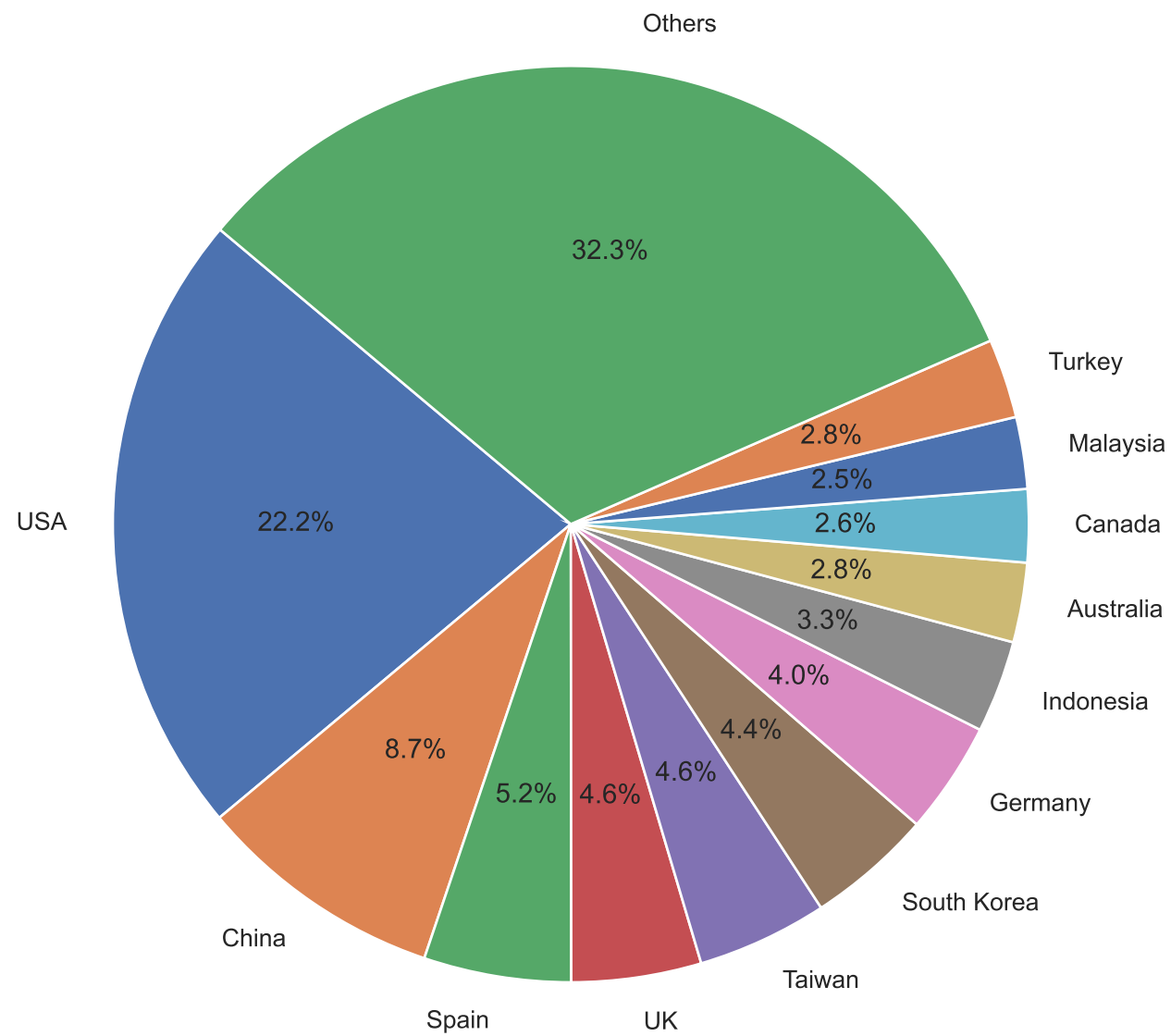
SCP (n=7,618)
