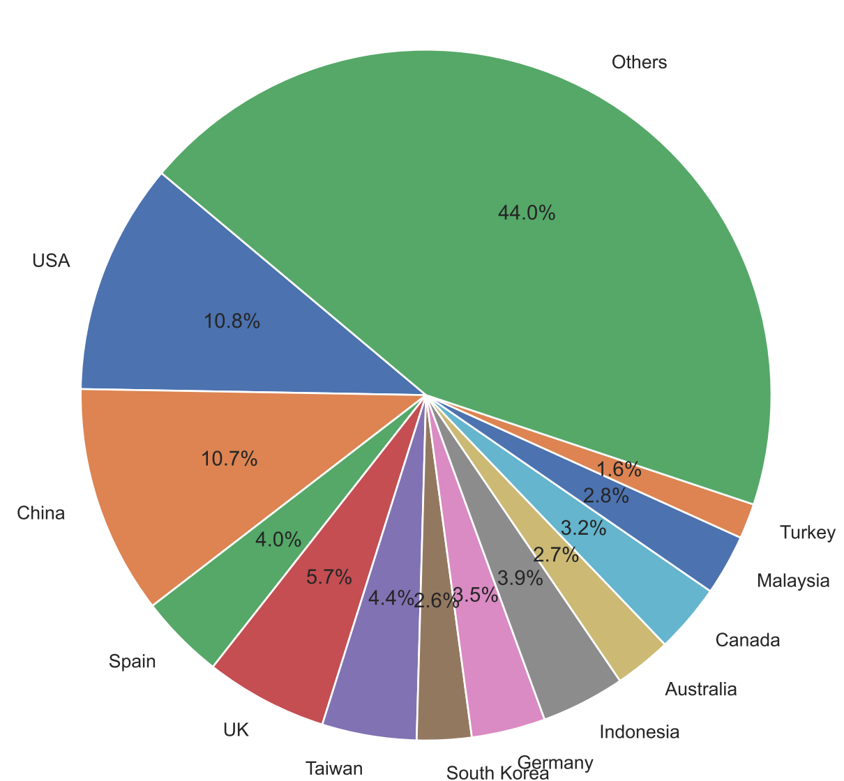
MCP (n=1,763)
