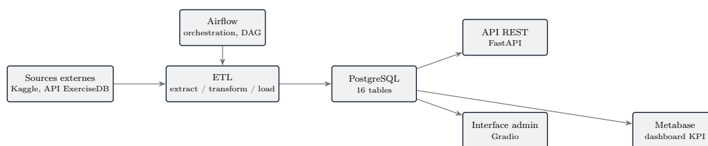
FIGURE 1 – Vue d'ensemble — l'ETL alimente PostgreSQL (orchestré par Airflow), consommé en aval par l'API REST, l'interface admin et Metabase. L'ensemble du périmètre est conteneurisé via docker compose (cf. §7).
