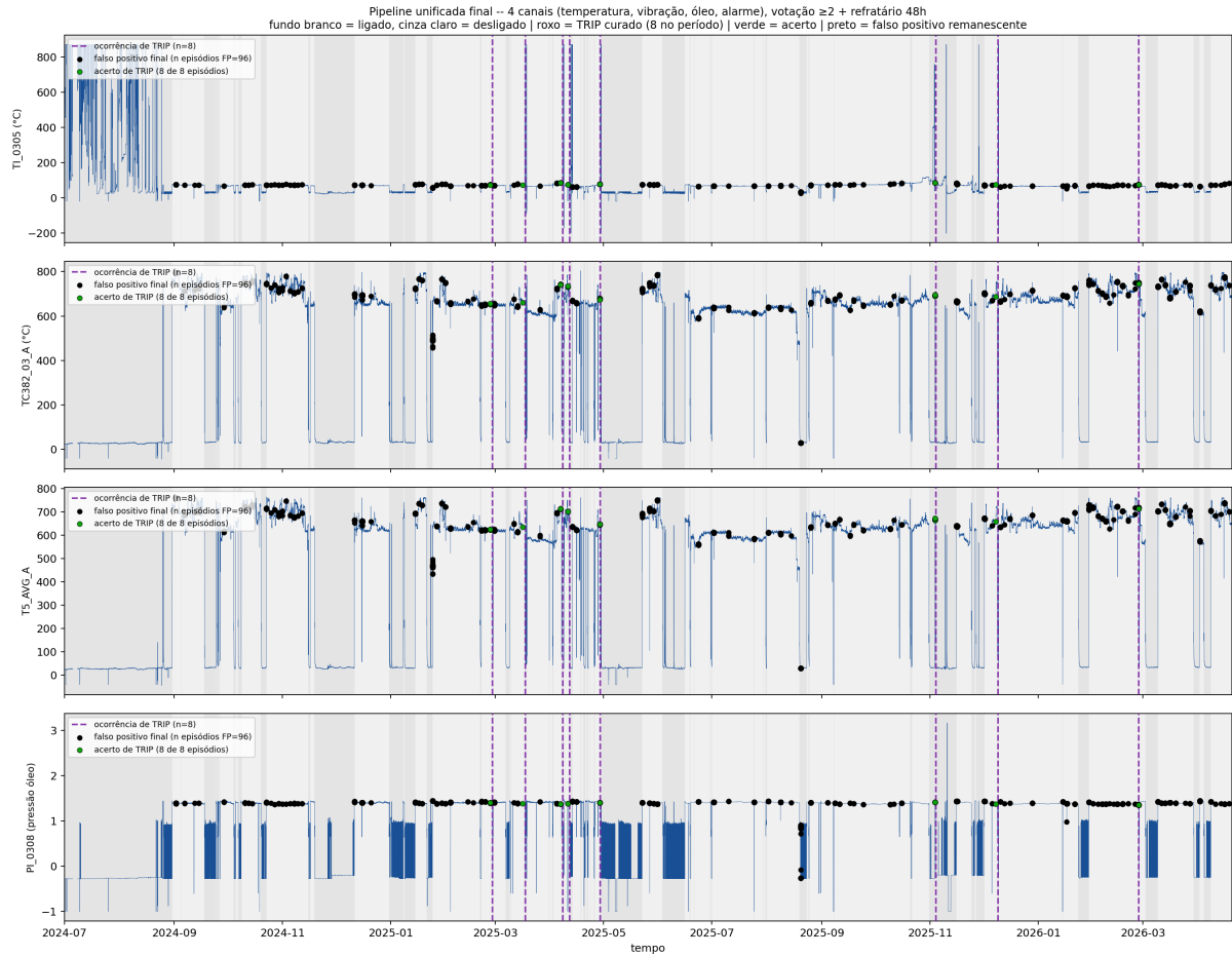
Figura 9: TI_0305 / TC382_03_A / T5_AVG_A / PI_0308 com a decisão final da pipeline unificada: roxo = TRIP curado (8 no período); verde = acerto (todos os 8); preto = falso positivo remanescente.
