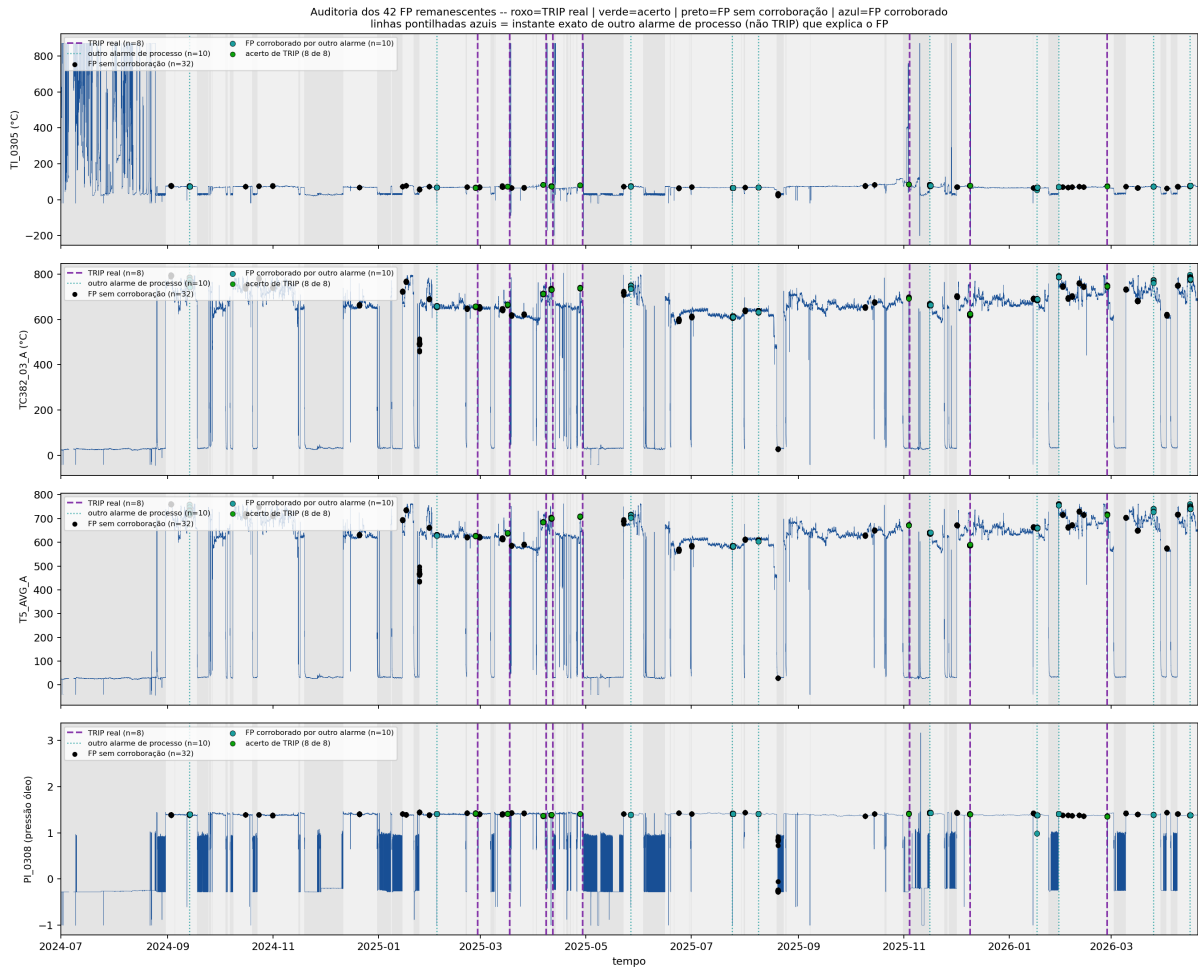
Figura 10: Série bruta completa com a auditoria dos 42 FP: roxo = TRIP real; verde = acerto; preto = FP sem corroboração por outro alarme; azul = FP corroborado; linhas pontilhadas azuis finas = instante exato do outro alarme de processo que explica cada FP corroborado.
