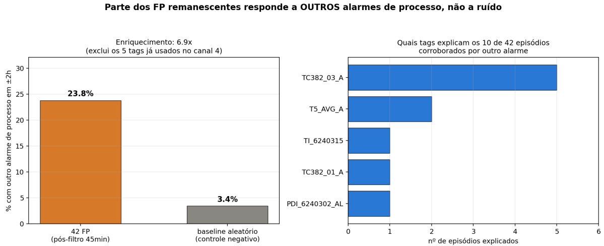
Figura 9: Esquerda: taxa de corroboração por outro alarme nos 42 FP vs. baseline aleatório (controle negativo). Direita: quais tags do catálogo explicam os 10 episódios corroborados – concentradas em alarmes do próprio sensor de temperatura de mancal (TC382_03_A, T5_AVG_A).
