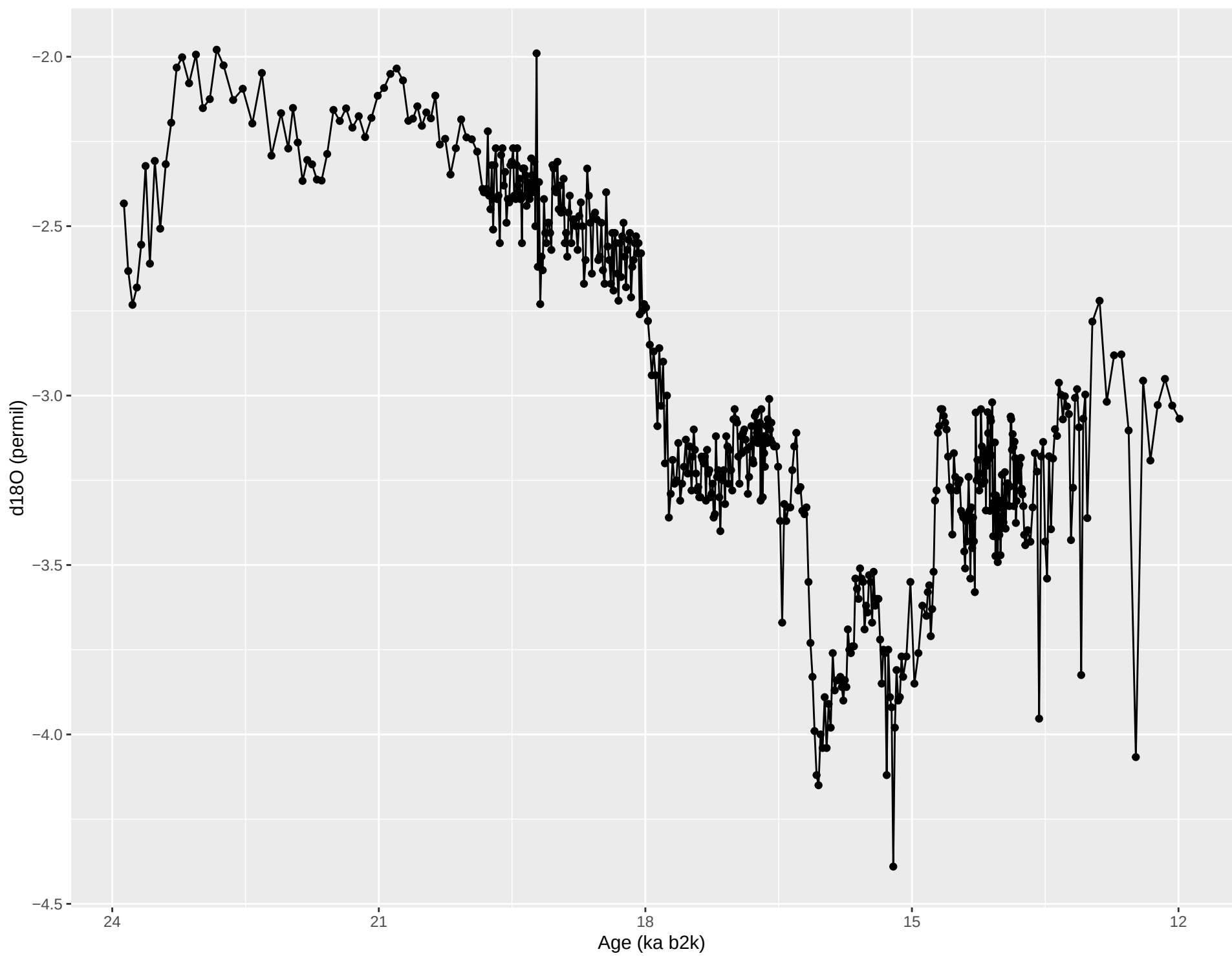
d18O vs age –Glas (Laura Endres)
