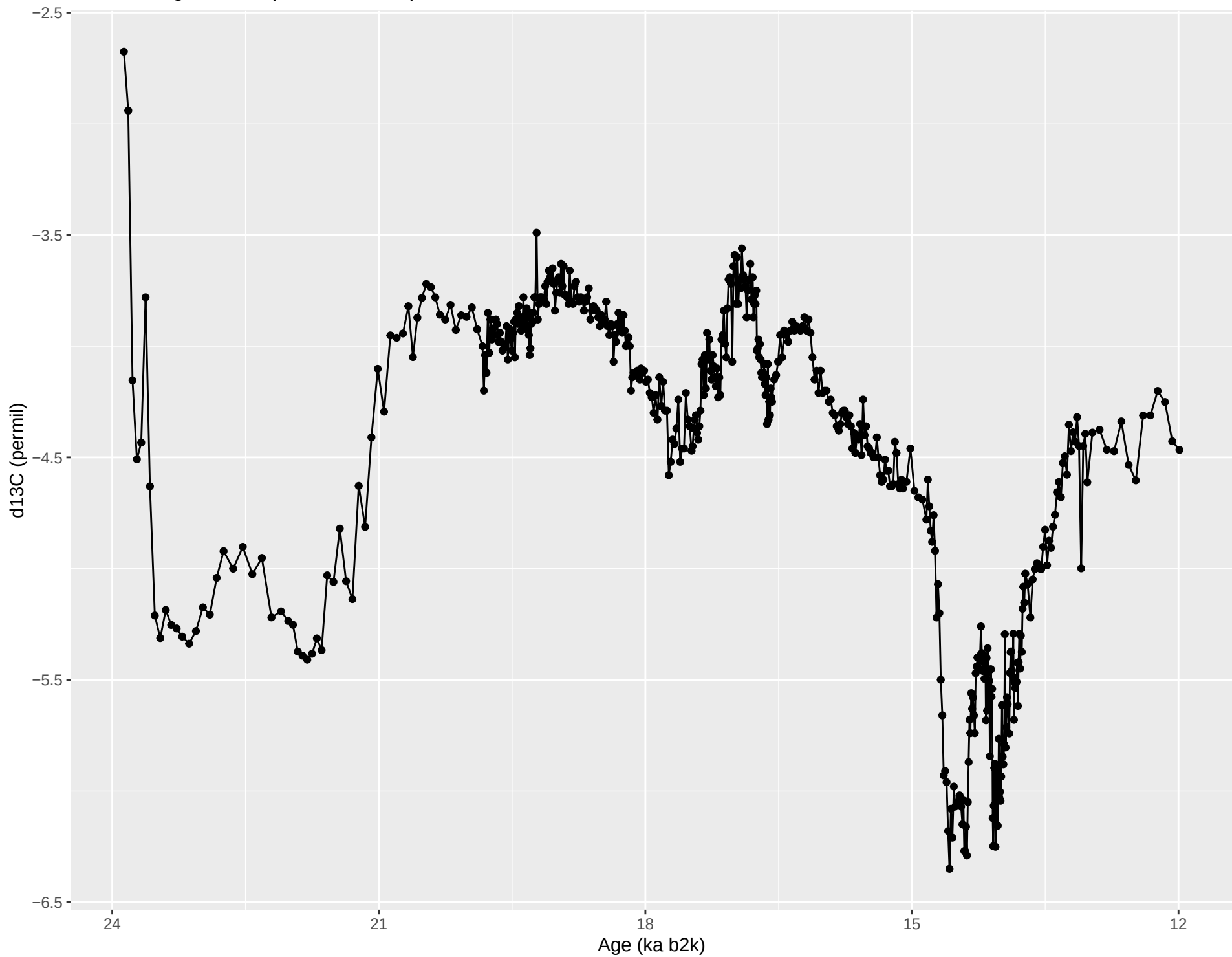
d13C vs age -Glas (Laura Endres)
