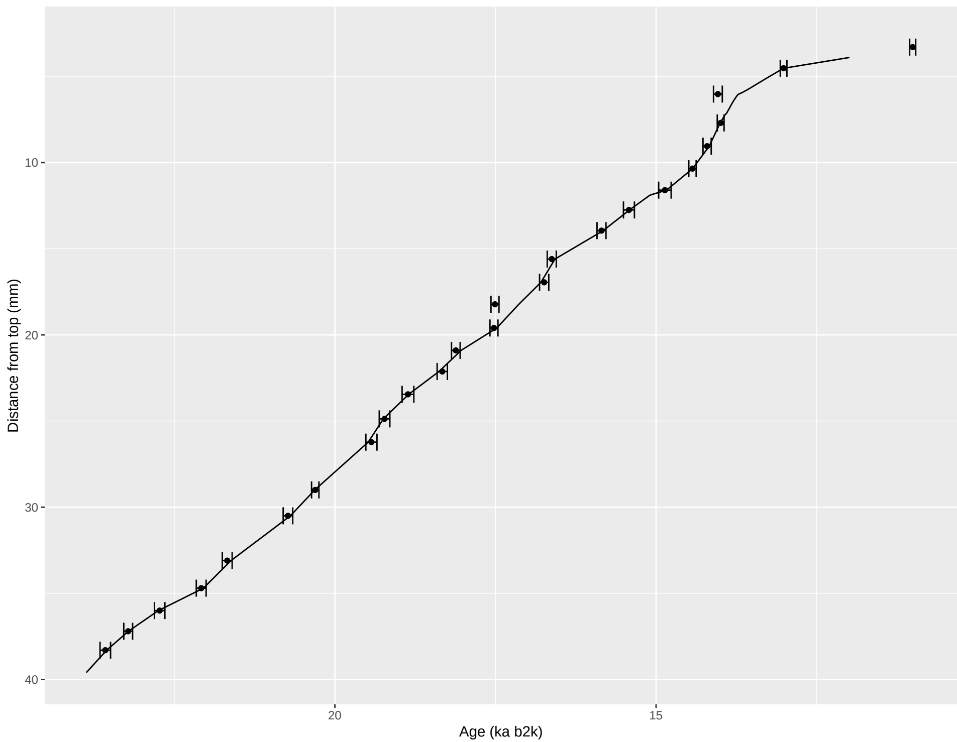
Age model: Glas (Laura Endres)
