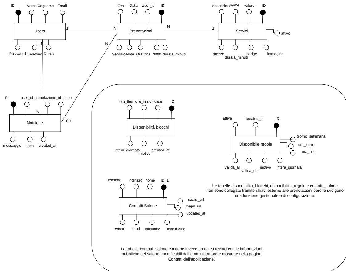
Figura 1: Diagramma Entità-Relazione.
