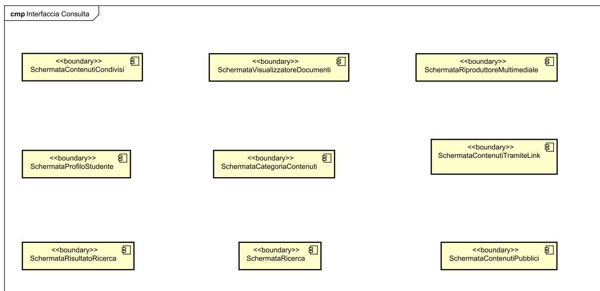
Figura 8: Interfaccia del sottosistema Consultazione
