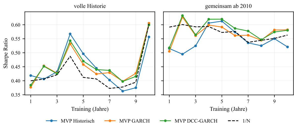
Abbildung 2: Sharpe Ratio über die Trainingsfenster, voller und gemeinsamer Bewertungszeitraum TRBC, Prognosehorizont 1 Tag, links die volle Historie des jeweiligen Fensters, rechts der für alle Fenster identische Zeitraum ab 01.01.2010.
